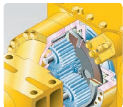
Nasse Lamellenbremsen
