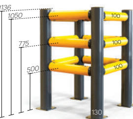
iFlexRail Ochrana sloupů Column Guard ***
