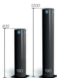
RackGuard Cold Storage Rack Chránič regálových stojin ***
