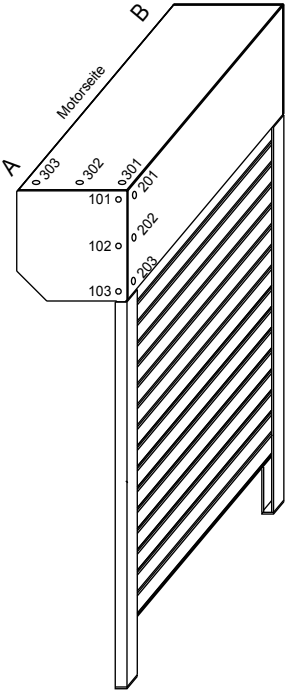
Kabelposition
