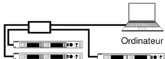
Routeur avec DHCP
