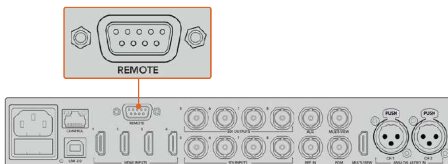
Connectez une caméra au mélangeur via le port RS-422 situé sur la face arrière.
