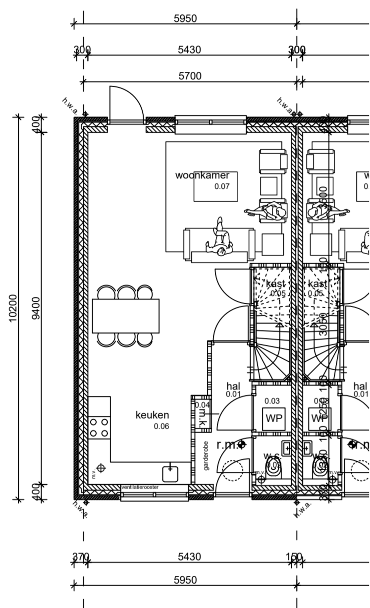
BEGANE GROND
