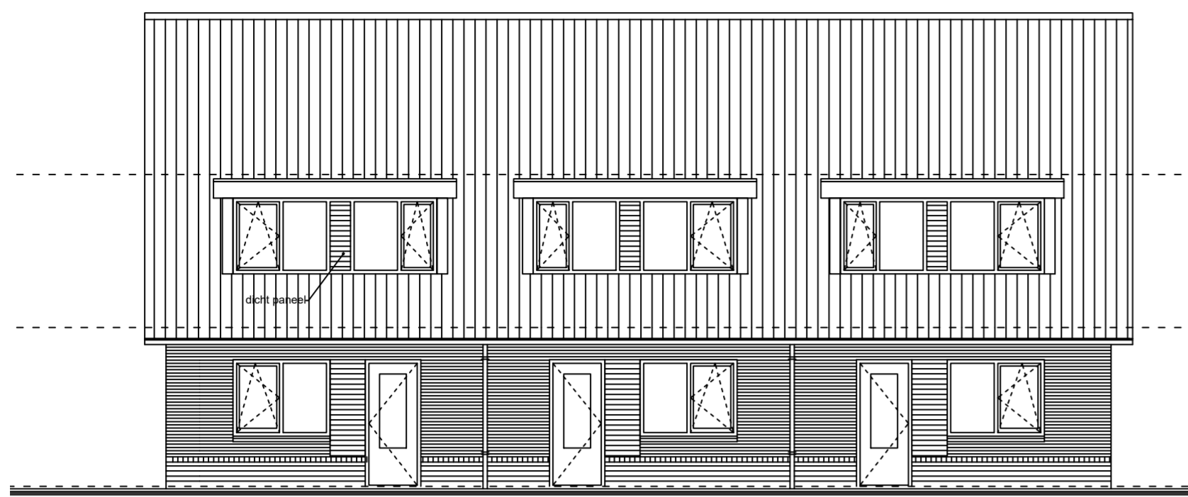
voorgevel
