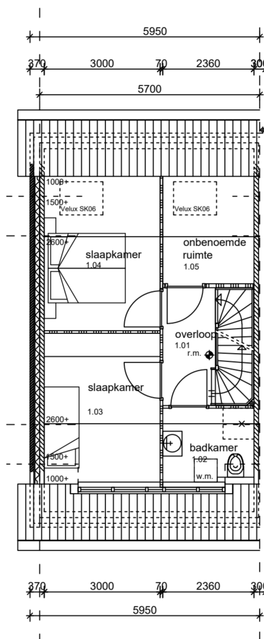
VERDIEPING
