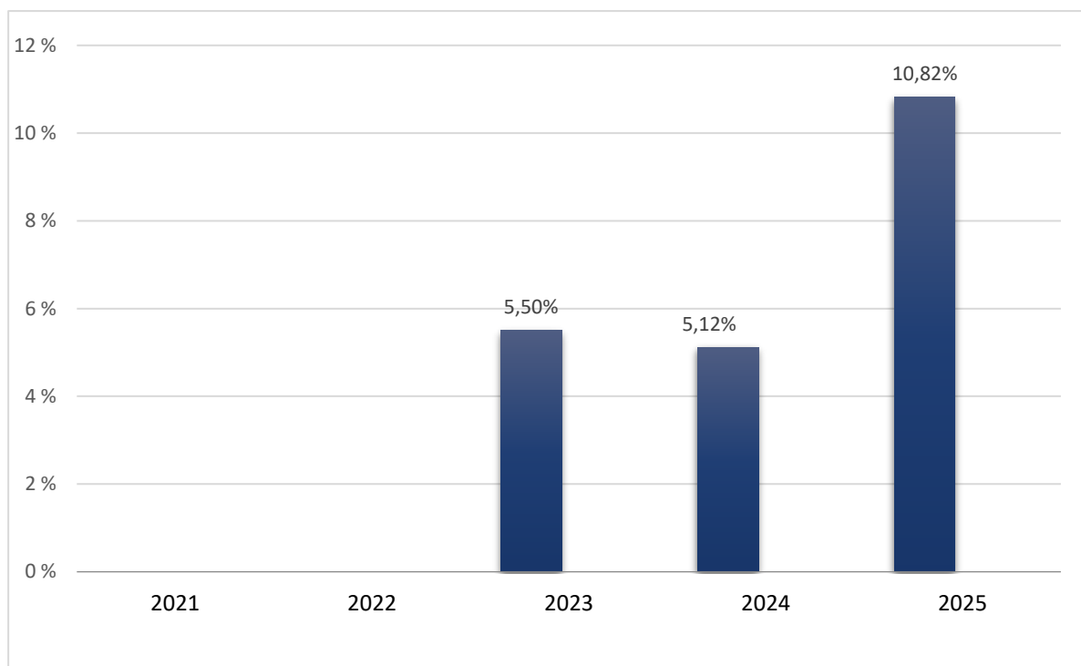
Graf výkonnosti investičních akcií (CZ0008049129) (v EUR)
