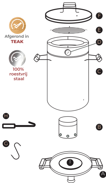
AFBEELDING. 1 HANDGRIEPSET BOVEN (CILINDER)
