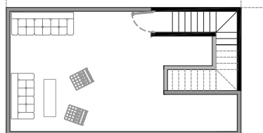
PLANTA ALTA.
