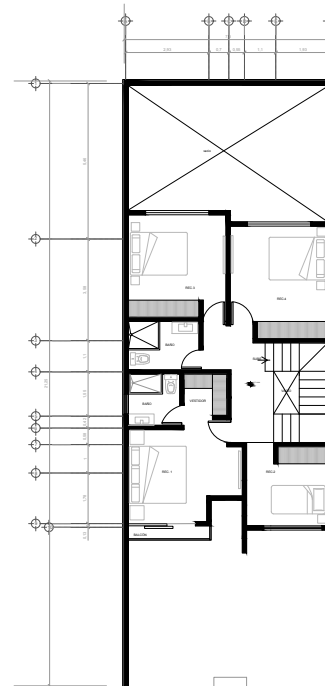
PRIMER PISO
