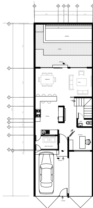
PLANTA BAJA
