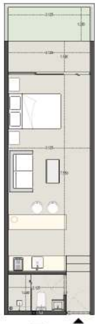
ESTUDIO GARDEN VISTA: FACHADA POSTERIOR AREA TOTAL: 38.40M 2 AREA VERDE: 3.59M 2
