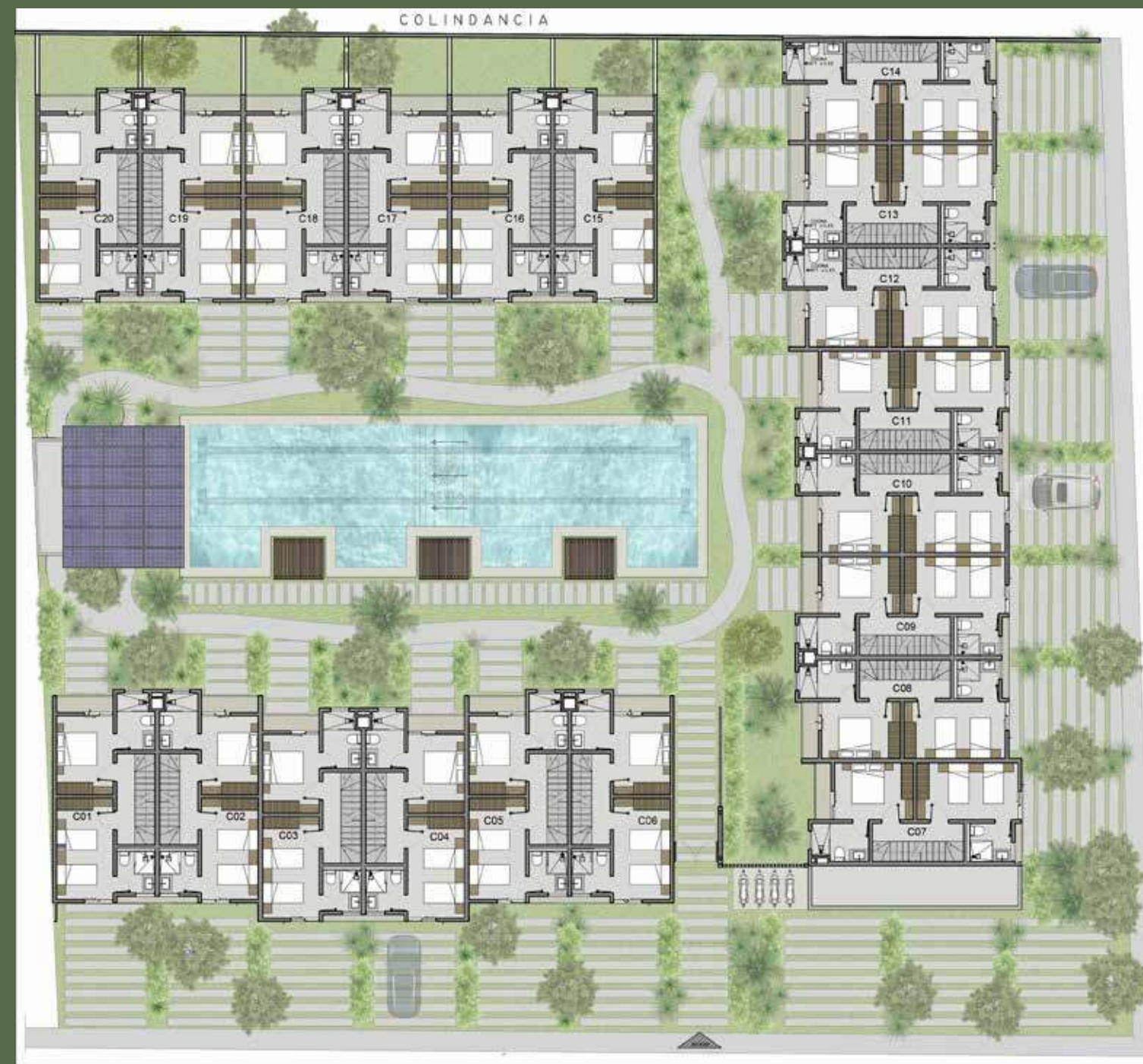
Primer nivel
