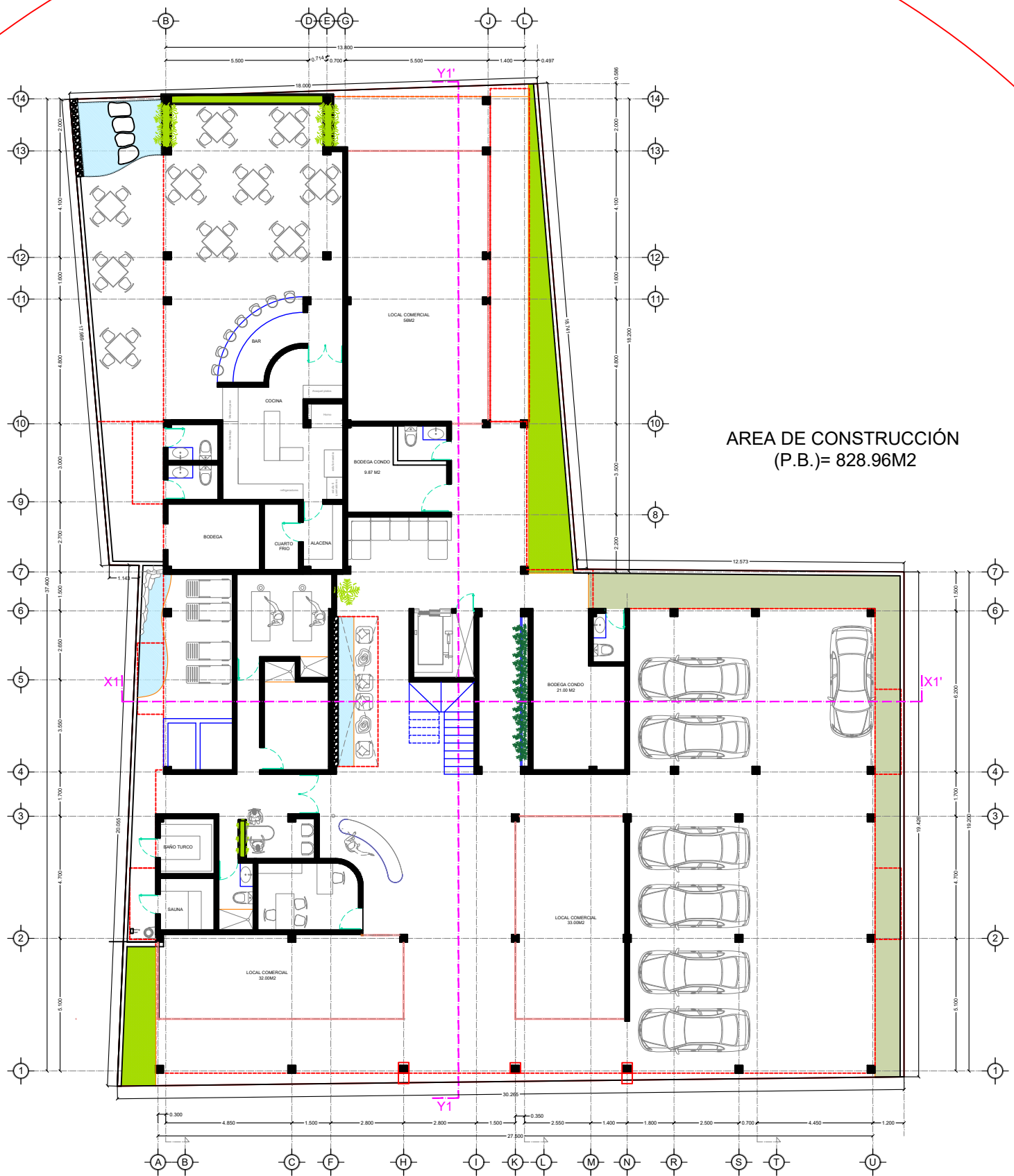
PLANTA ARQUITECTONICA PLANTA BAJA real ejecutiva
