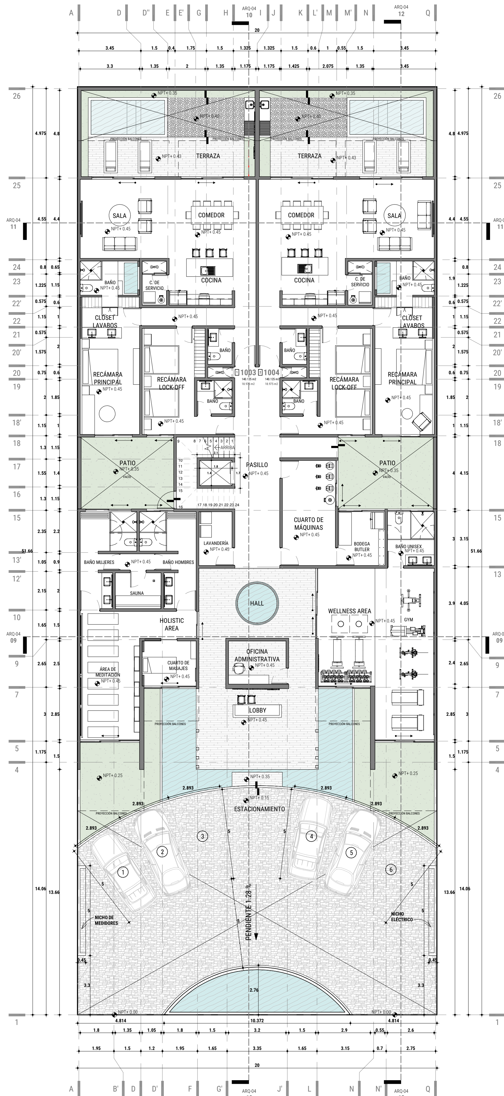
02 PLANTA BAJA ARQUITECTÓNICA ESC: 1 : 125
