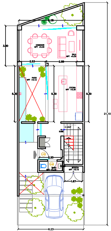
1 PLANTA ARQ. BAJA ESC. 1:50 ACOTACIÓN m
