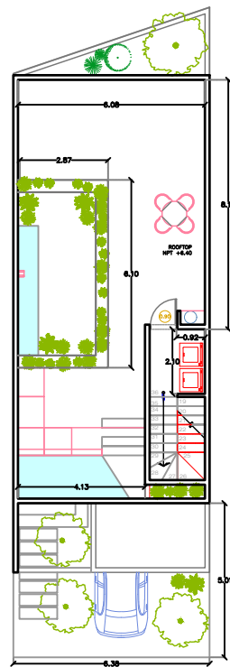
3 ROOF TOP ESC. 1:50 ACOTACIÓN m
