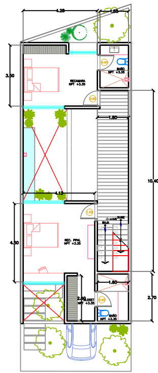
2 PLANTA ARQ. ALTA ESC. 1:50 ACOTACIÓN m
