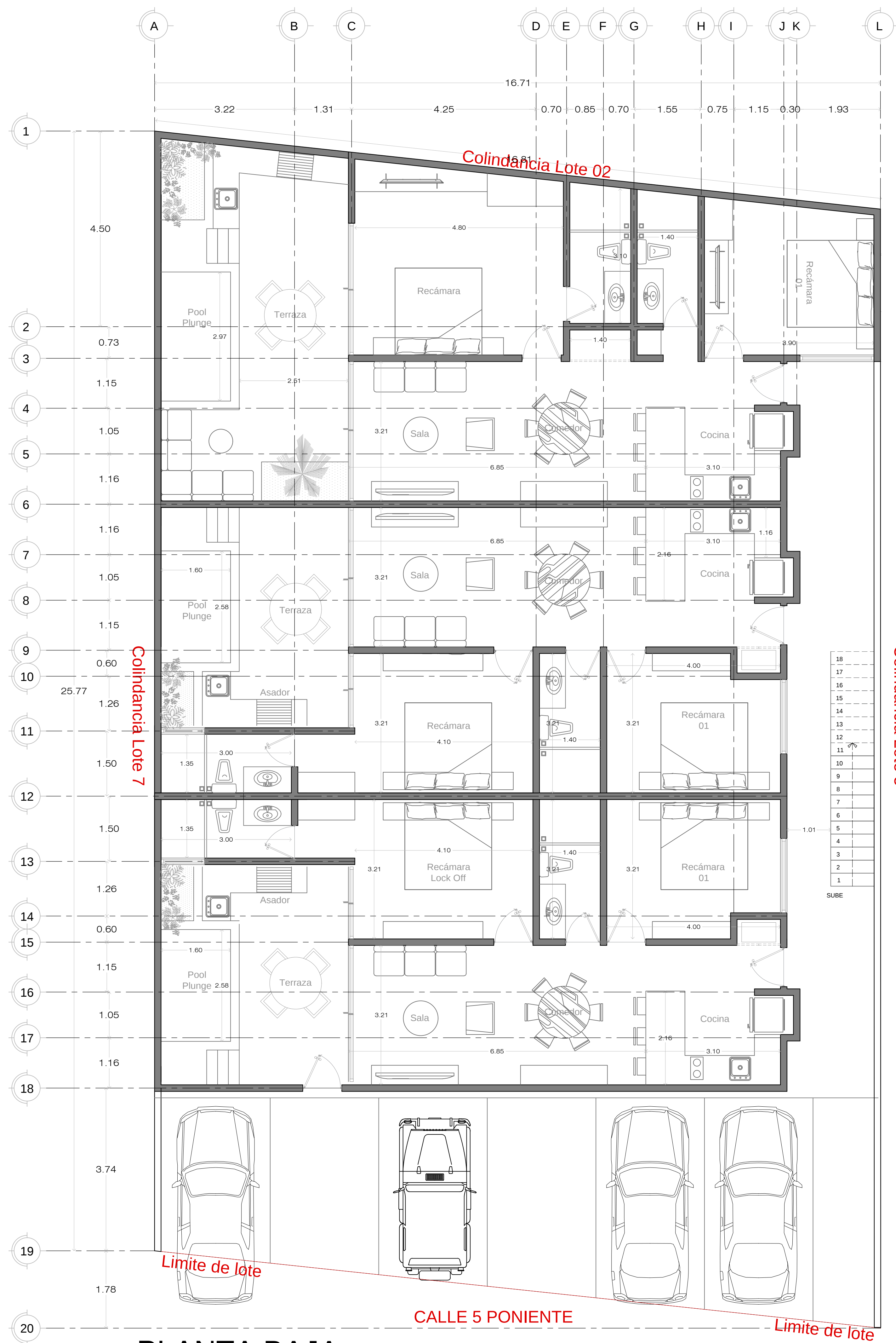
PLANTA BAJA
