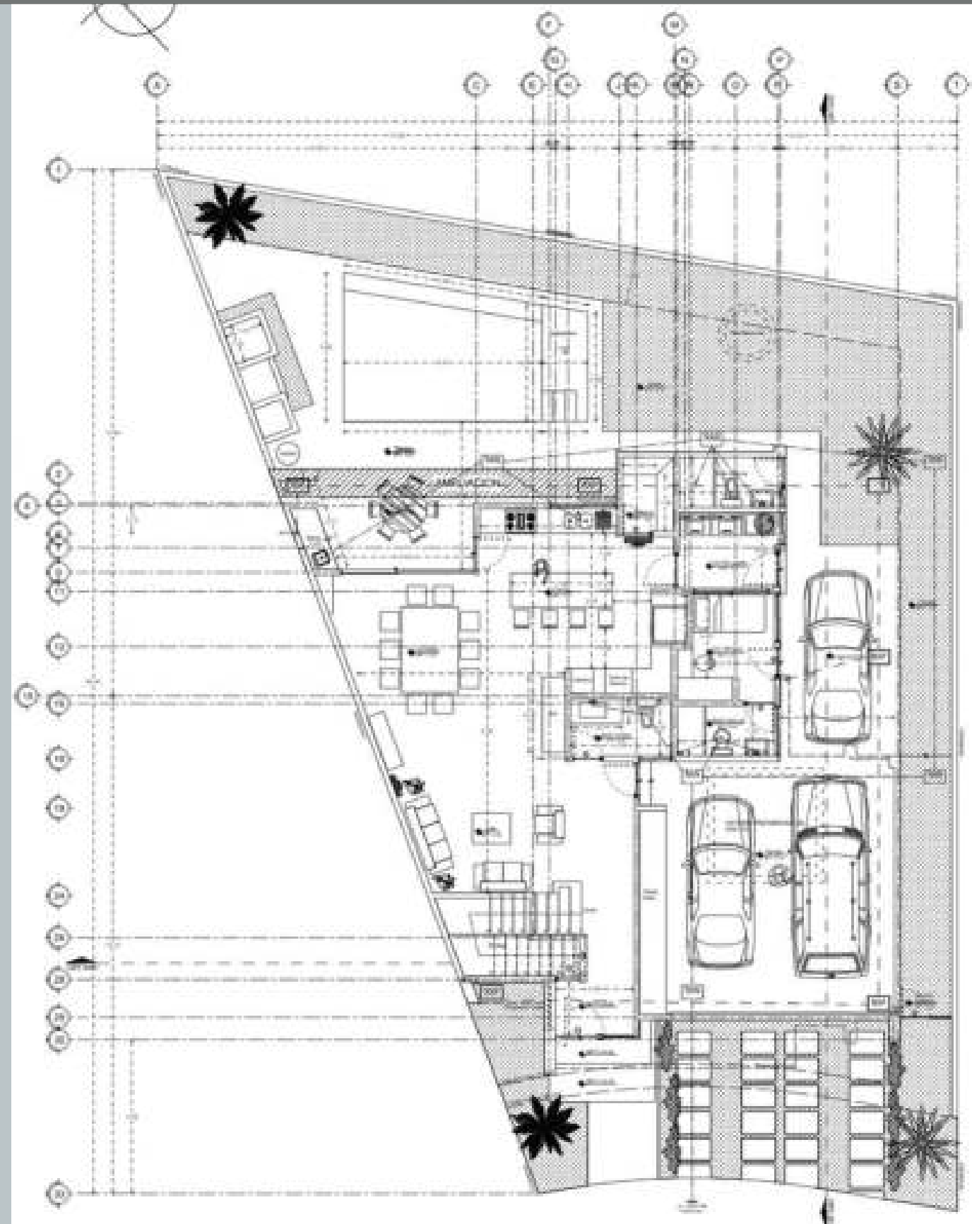
Planta Baja 169.52 m2
