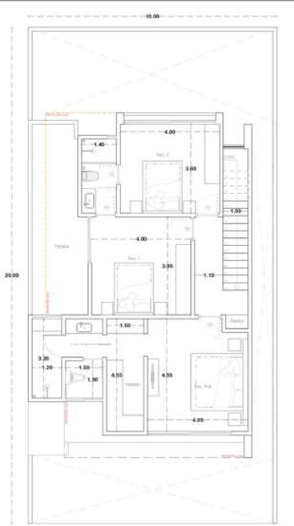
PLANTA ALTA 115 M2
