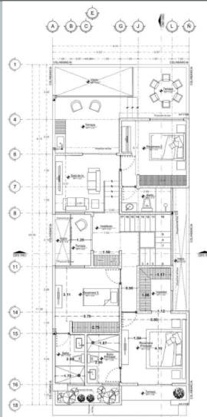
PLANTA ALTA 122.54 m2
