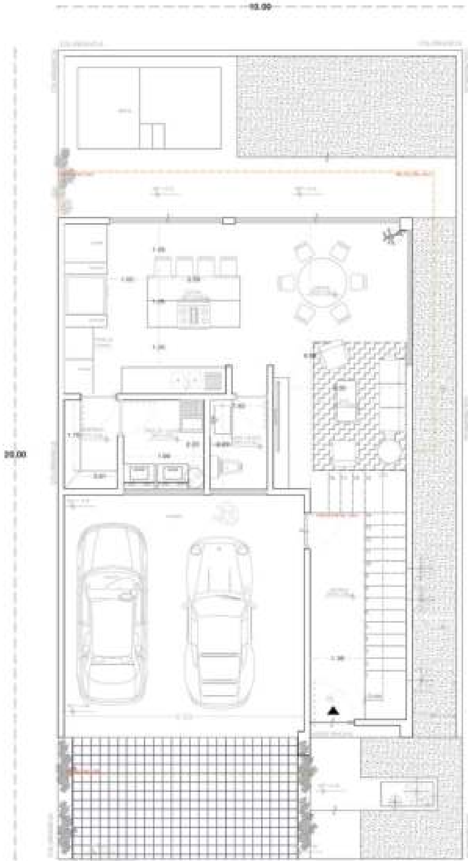
PLANTA BAJA 132 M2
