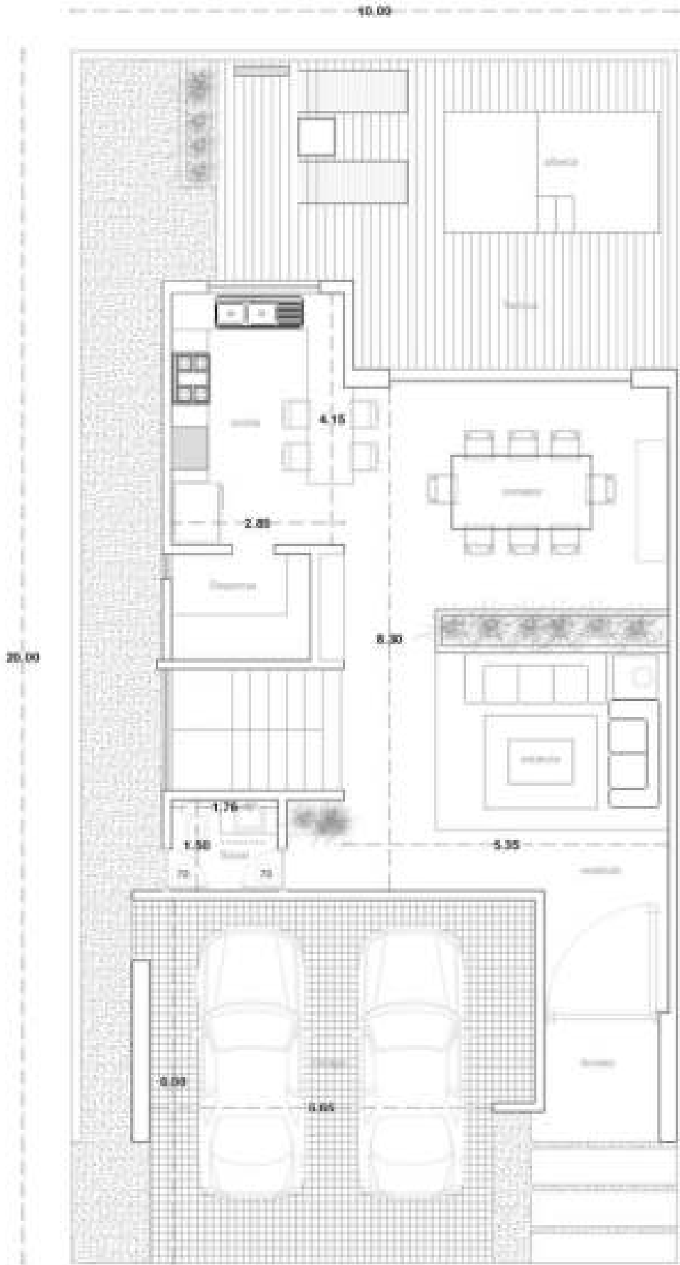
PLANTA BAJA 126 M2
