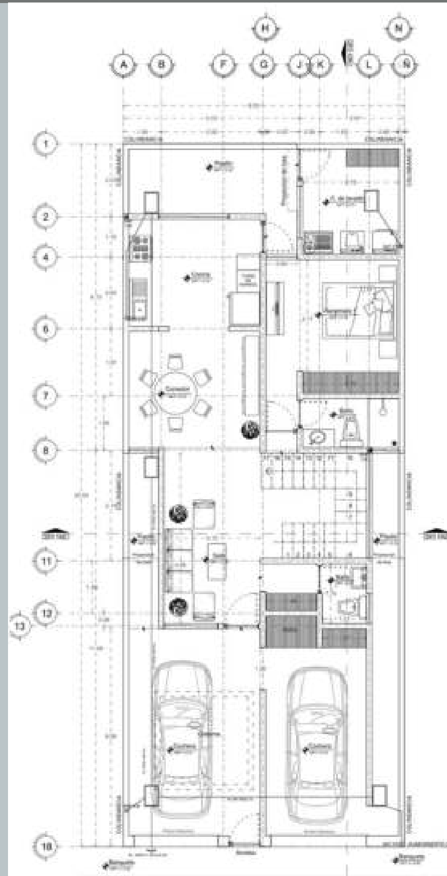
PLANTA BAJA 139.48 m2
