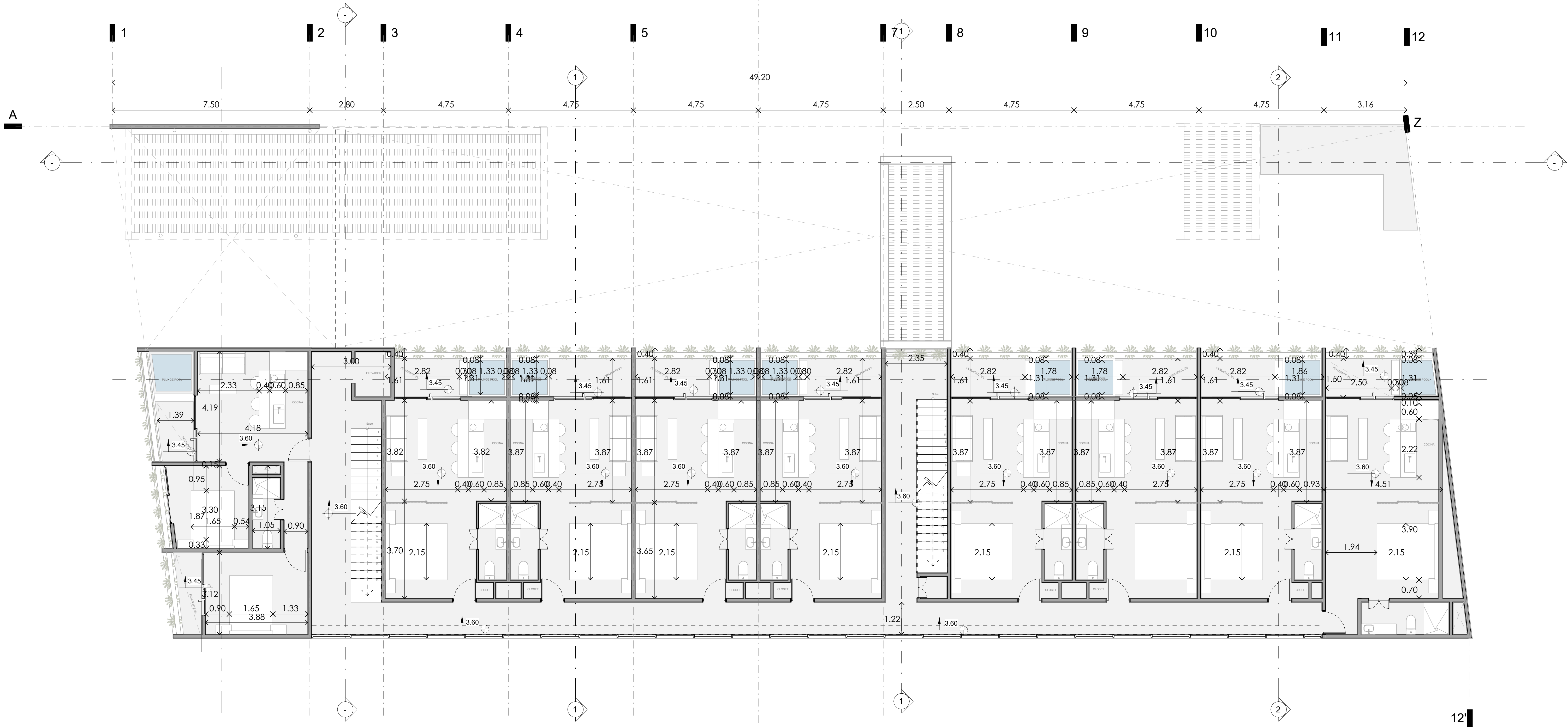
2 ARQ02. Nivel 02 1:75
