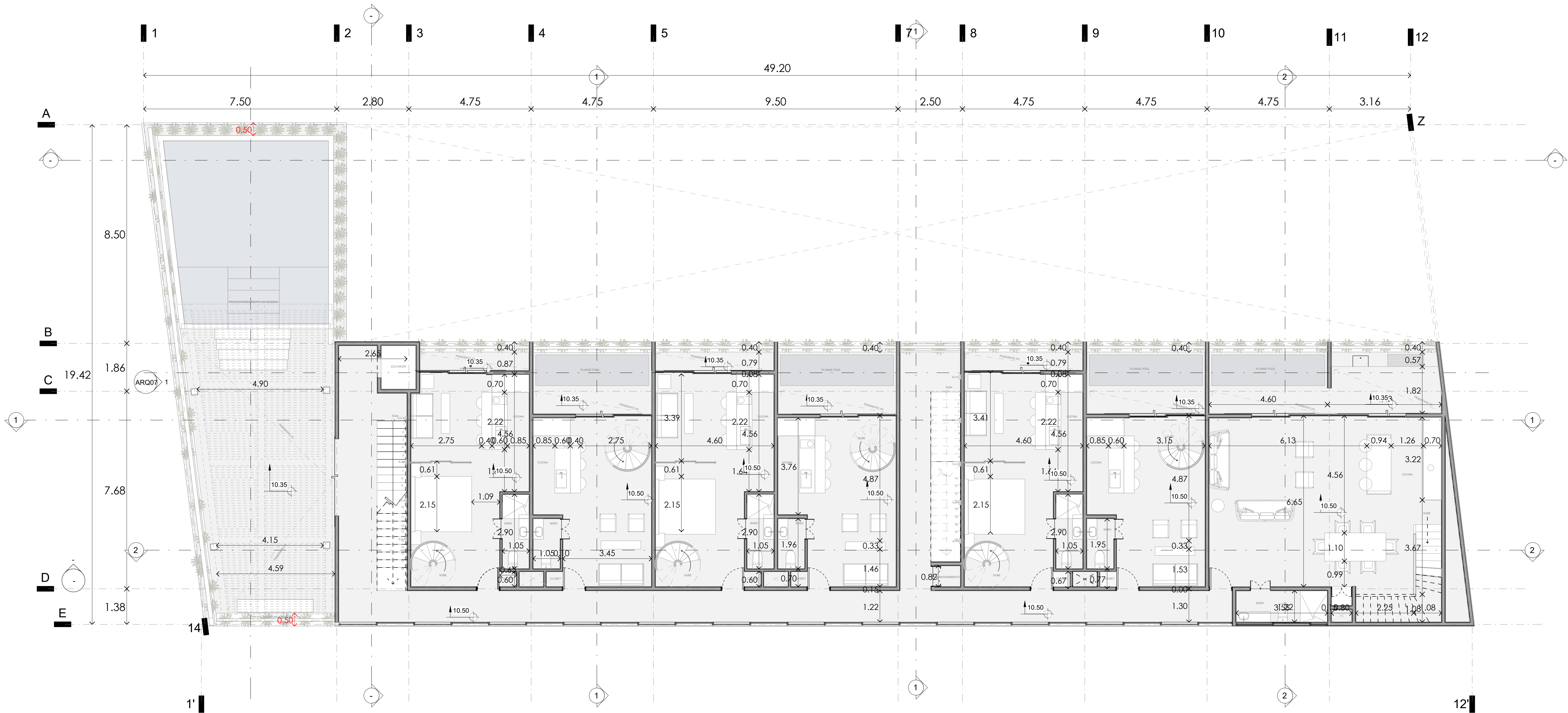
4 ARQ04. Nivel 04 1:75
