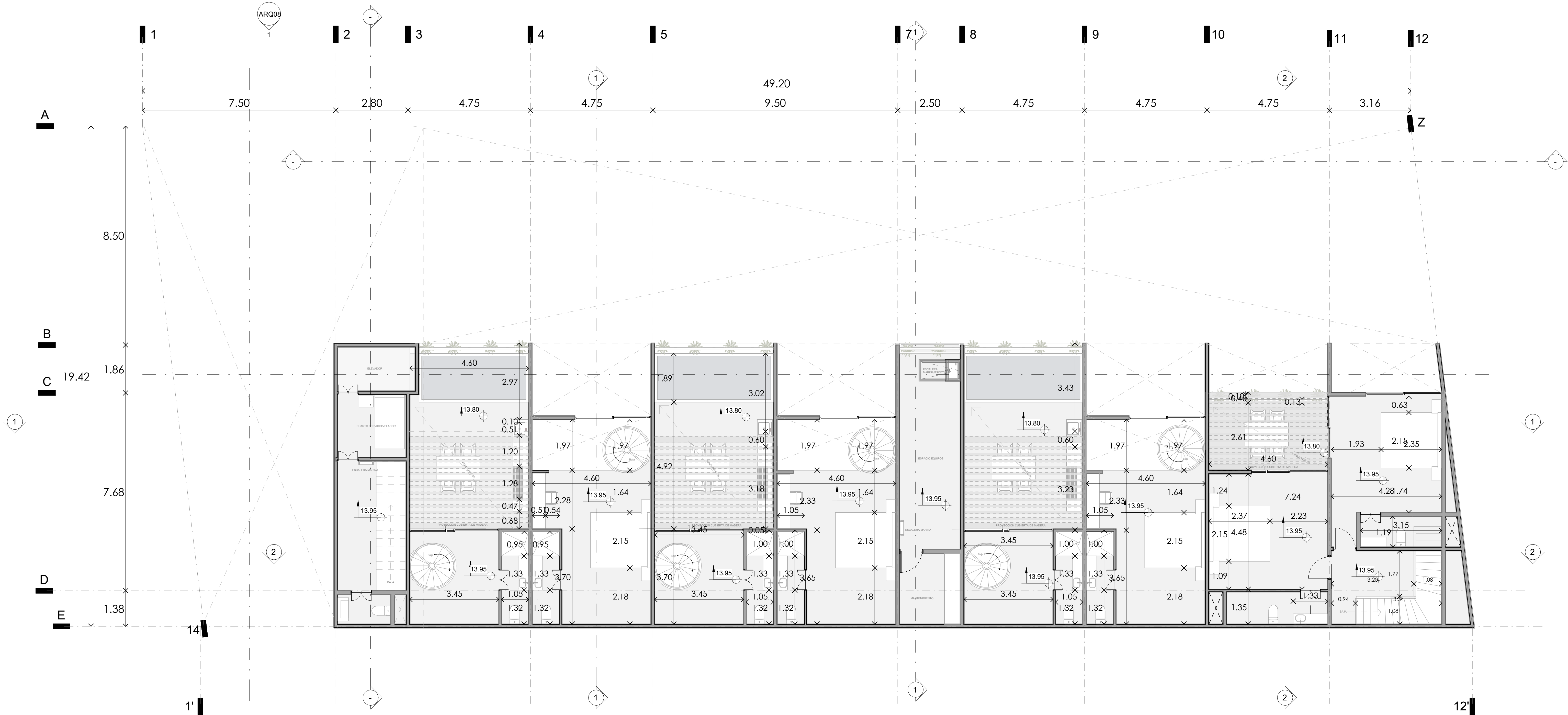
1 ARQ05. Nivel 05 1 : 75
