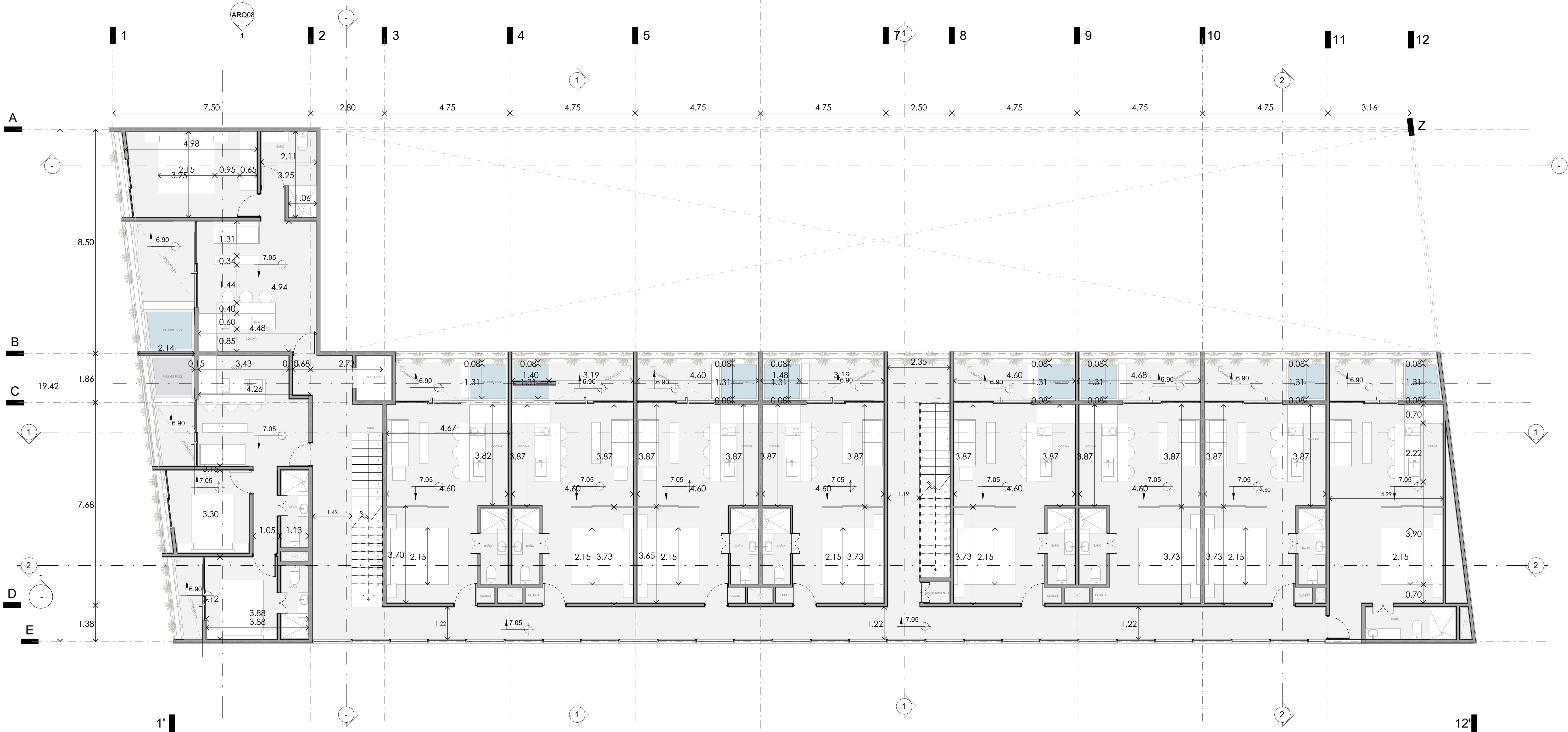
3 ARQ03. Nivel 03 1 : 75
