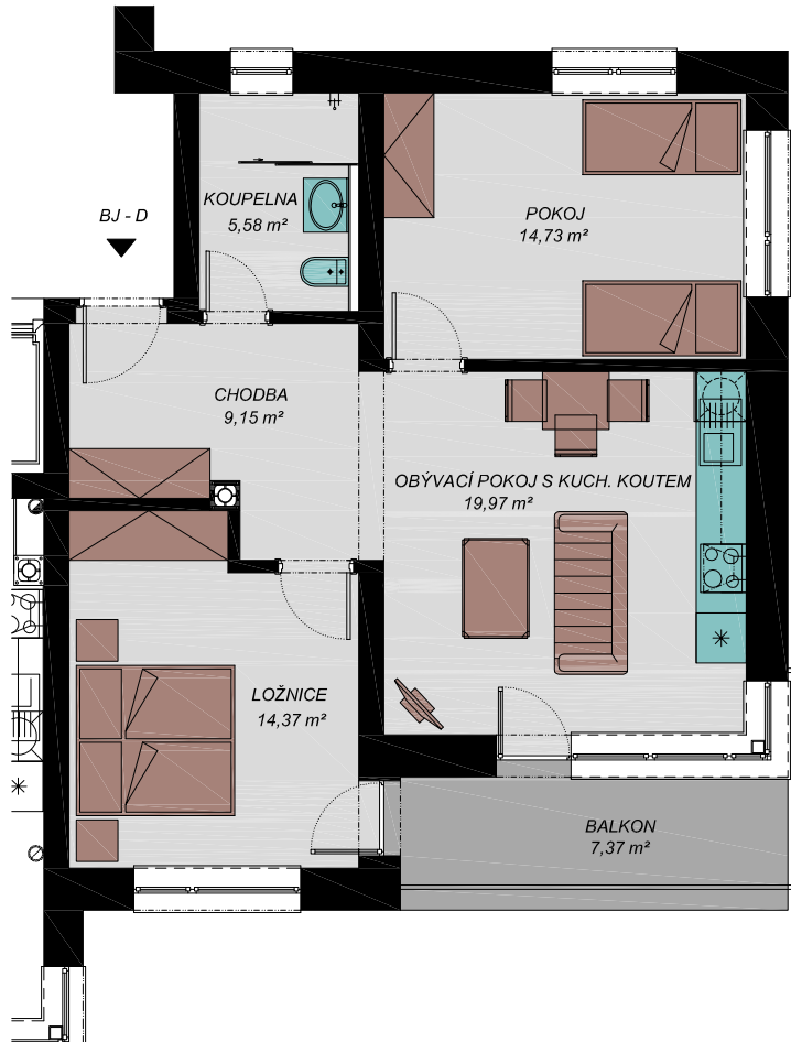
Bytová jednotka D - 63,80 m 2
