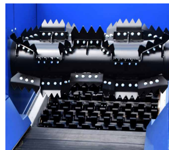
Dosing Rotor
