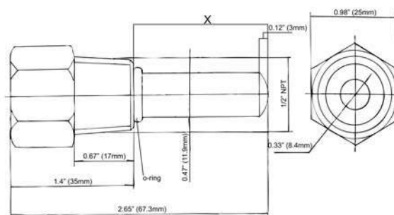
1/2" TST050
