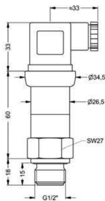
G1/2" DIN 3852 with ISO 4400
