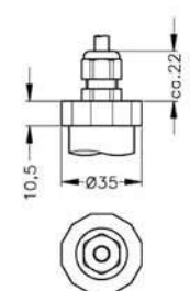
Cable gland (IP 67) 5,6
