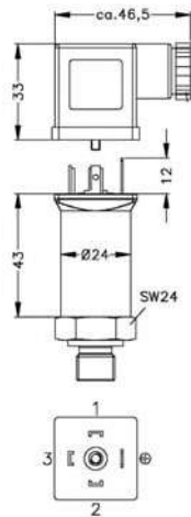
ISO 4400 (IP 65)
