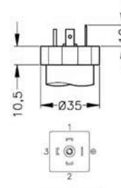
DIN 43650 A 1/2" NPTF conduit fitting
