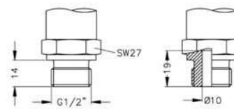
G1/2" open port DIN 3852; M20x1.5
