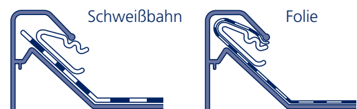
Zweiteiliger Dachrandabschluss
