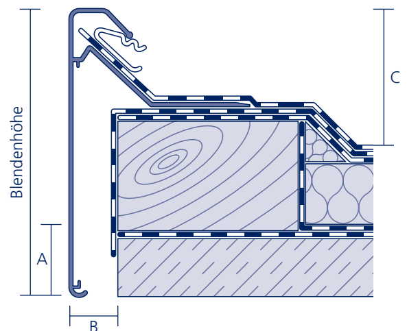
Zweiteiliger Dachrandabschluss
