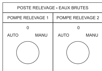
Étiquette de façade d'armoire
