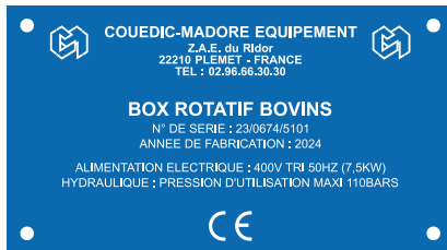
Plaque constructeur en PVC
