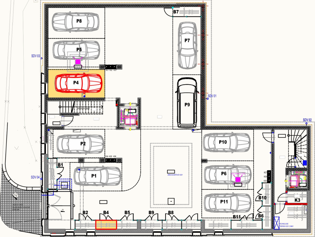
PRVNÍ PODZEMNÍ PODLAŽÍ - GARÁŽE
