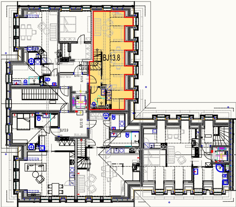
TŘETÍ NADZEMNÍ PODLAŽÍ
