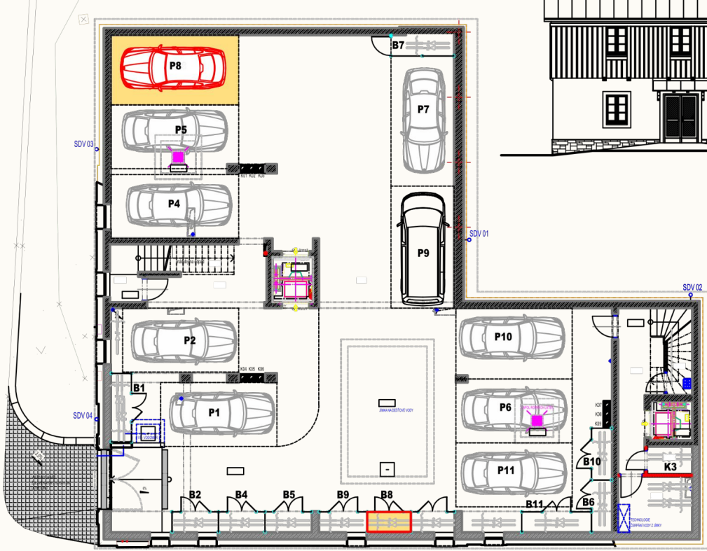
PRVNÍ PODZEMNÍ PODLAŽÍ - GARÁŽE
