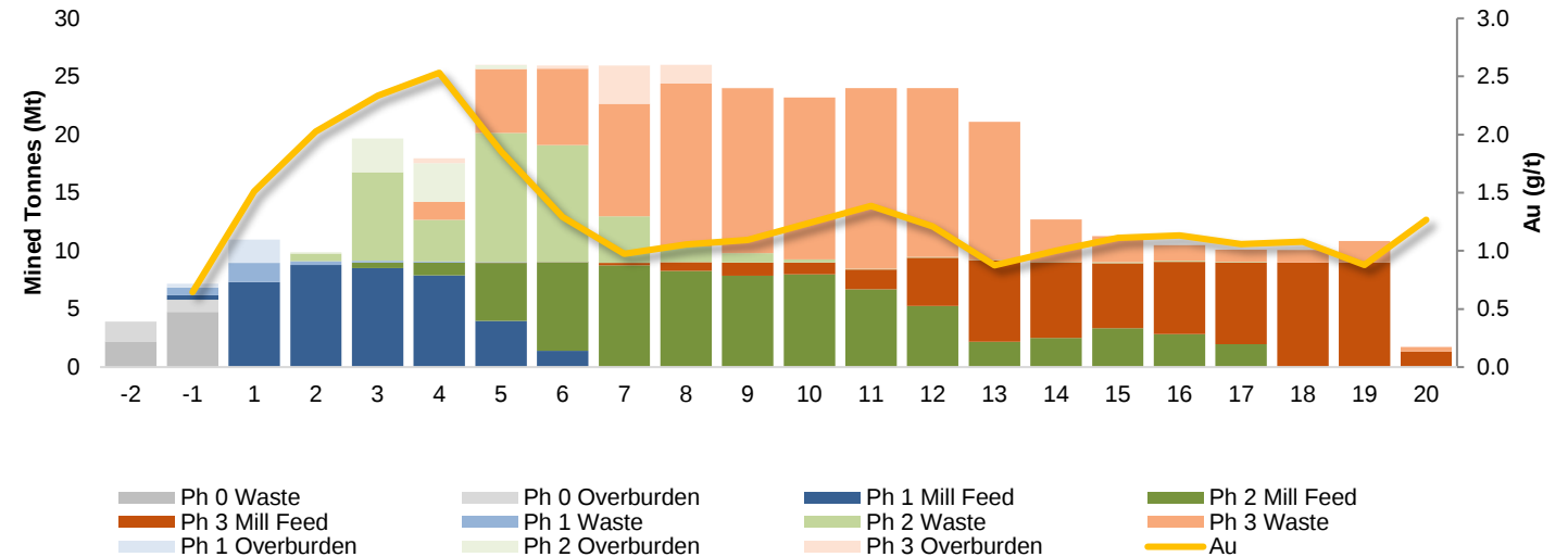
Production Schedule: 9.0 Mtpa / 25 ktpd
