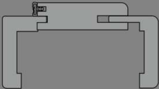
ZARGE MIT RUNDKANTE CHÂSSIS AVEC CHANTS ARRONDIS
