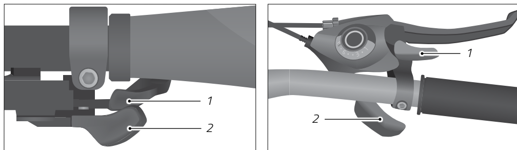
Fig.: Unità di comando sul manubrio per l'innesto di pignoni e corone (esempio del lato destro del manubrio)
