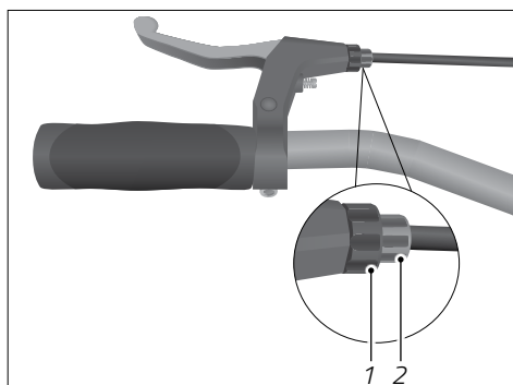
Fig.: Posizione controdamo e vite zigrinata (esempio)
