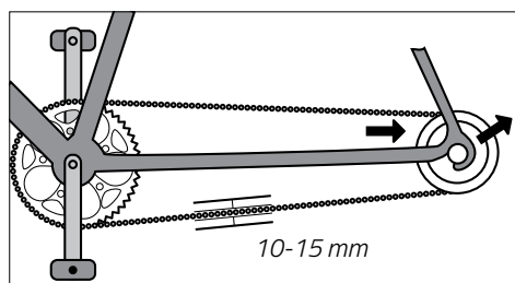
Fig.: Tensione della catena (esempio)
