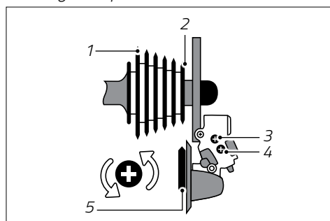
Fig.: Schema di deragliatore (esempio)
