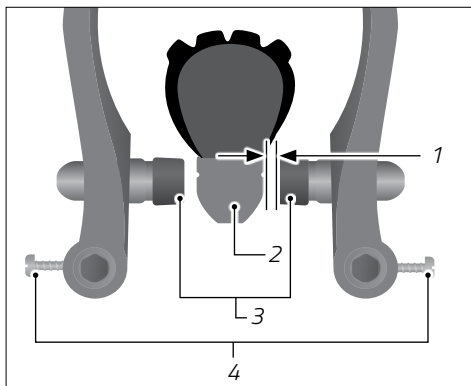
Fig.: Distanza pattino del freno (esempio)
