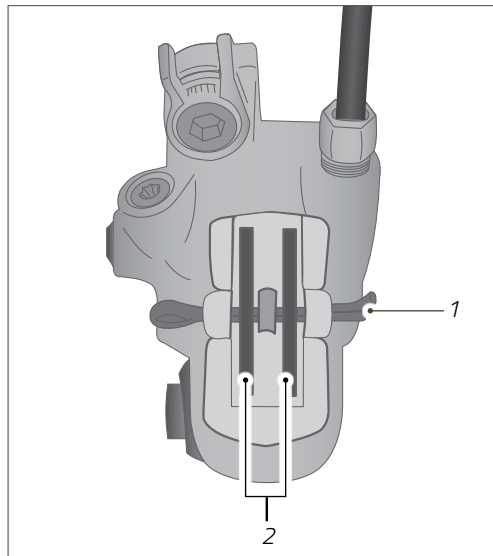
Fig.: Pinza del freno con splint (esempio)
