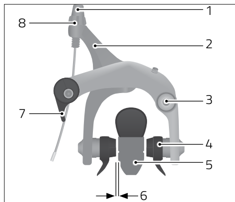
Fig.: Freno a pinza bicicletta da corsa (esempio)
