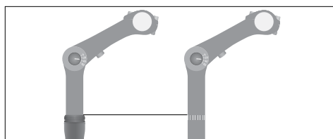
Fig.: Marcatura della profondità minima di inserimento in attacco a tubo con incastro interno (esempio)
