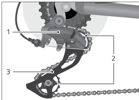
Fig.: Componenti mobili di un deragliatore (esempio)
