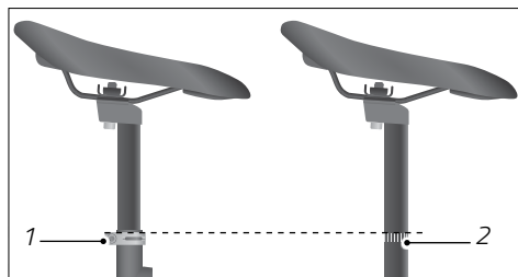
Fig.: Profondità minima di inserimento del reggisella (esempio)
