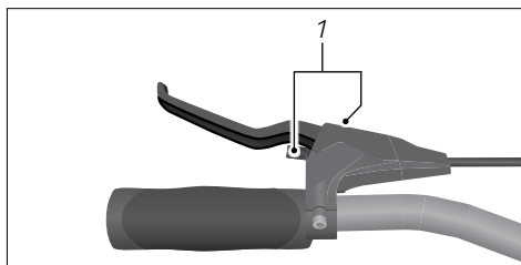
Fig.: Posizione della vite di regolazione (esempio)
