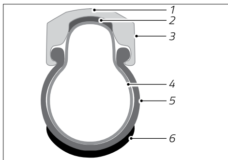
Fig.: Sezione di ruota con pneumatico (esempio)
