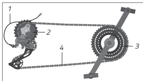
Fig.: Componenti di un deragliatore (esempio)
