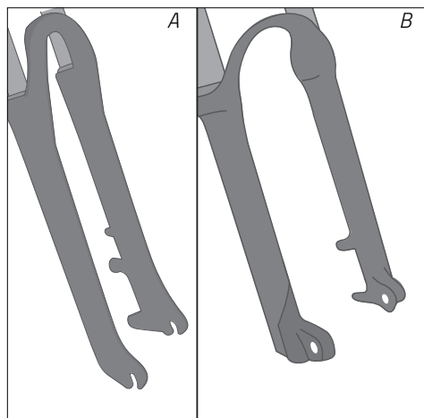
Fig.: Forcellini aperti (A) e chiusi (B) (esempio)
