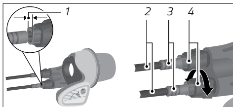
Fig.: Gioco della guaina del cavo (sin.) e vite di regolazione (dx.) (esempio)
