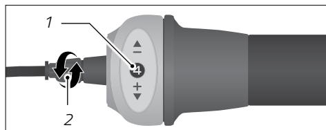
Fig.: Vite di regolazione su manopola del cambio (esempio)
