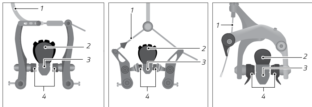
Fig.: Freni a pinza meccanici (esempio)
