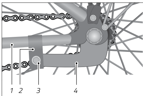
Fig.: Freno a contropedale (esempio)
