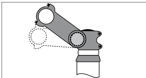
Fig.: Regolazione dell'inclinazione (esempio)
