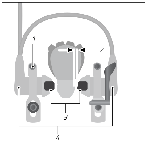
Fig.: Freno a pinza idraulico (esempio)
