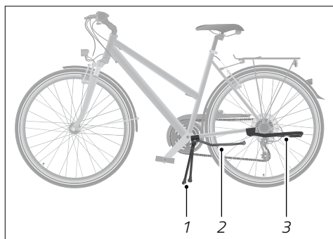
Fig.: Tipi di cavalletto (esempio)
