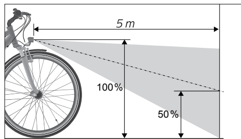
Fig.: Regolazione del fanale anteriore (esempio)
