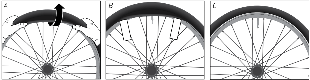
Fig.: Montaggio pneumatici rigidi o pieghevoli (esempio)
