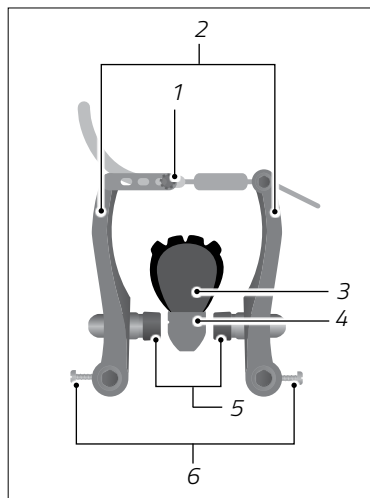
Fig.: Freno a pinza con passacavo (esempio)
