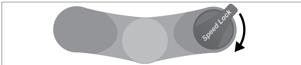
Fig.: Azionamento del lock-out sulla forcella ammortizzata (veduta dall'alto, esempio).
