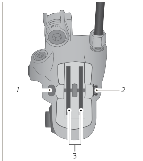
Fig.: Pinza del freno con vite (esempio)
