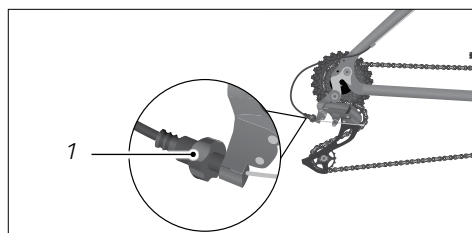
Fig.: Regolazione del deragliatore posteriore (esempio)
