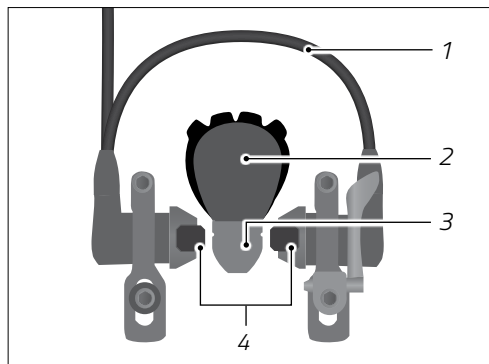
Fig.: Freno a pinza idraulico (esempio)
