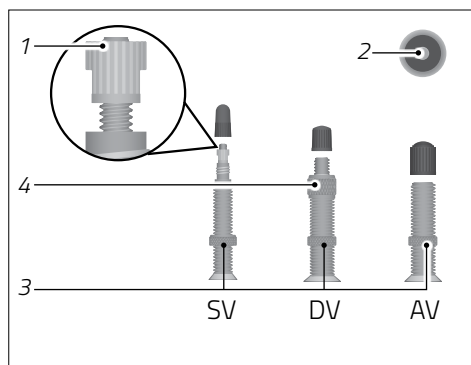
Fig.: Tipi di valvole (esempio)
