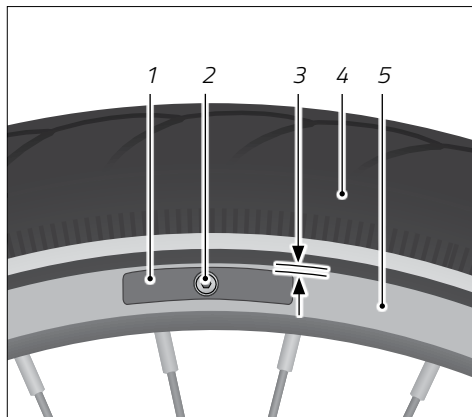
Fig.: Orientamento pattino del freno (esempio)
