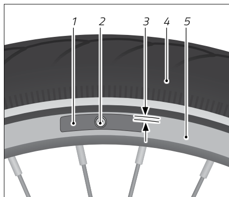
Fig.: Orientamento pattino del freno (esempio)
