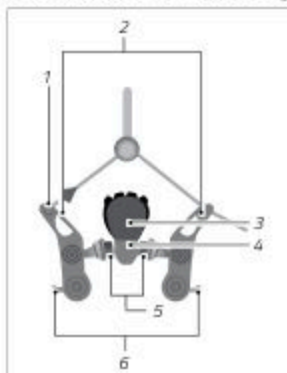
III: Fælgbremse med wirenippel (eksempel)
