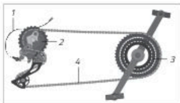
III.: Komponenter af et kædegear (eksempel)
