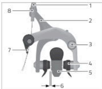
III: Fælgbremse racercykel (eksempel)
