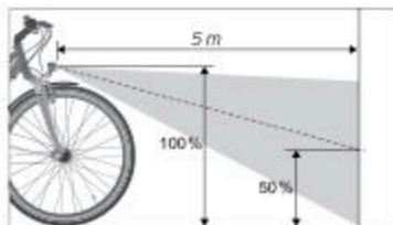
Ill.: Indstil forlygter (eksempel)
