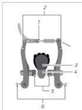
III: Fælgbremse med trækføring (eksempel)
