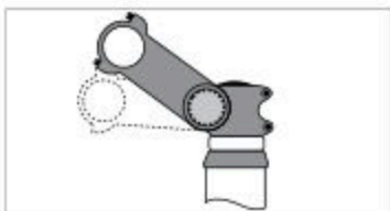
III.: Hældningsjustering (eksempel)
