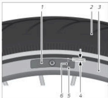
Ill: Bremsebelægning med skrue eller tap (eksempel)
