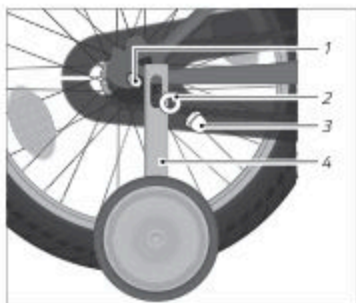
Ill.: Monter støttehjulet (eksempel)
