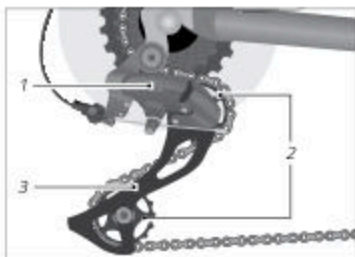
Ill.: Bevægelige komponenter af et kædegear (eksempel)
