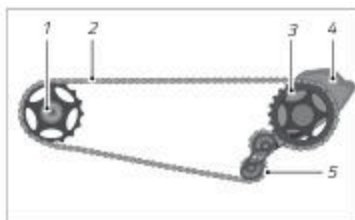
Ill.: Pinion-gear med kædedrev (eksempel)
