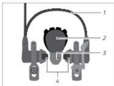
III: Hydraulisk fælgbremse (eksempel)
