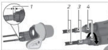
Ill.: Gearyderkablets slør (venstre) og indstillingsskrue (højre) (eksempel)
