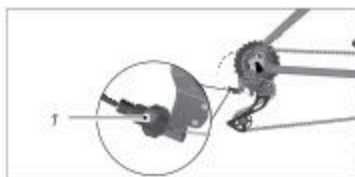
Ill.: Indstilling af bagskifteren (eksempel)
