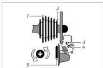
Ill.: Visning af en bagskifter (eksempel)
