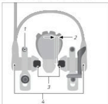
III: Hydraulisk fælgbremse (eksempel)
