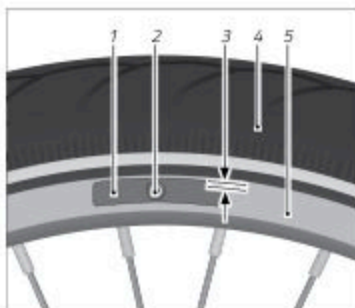
III: Justering bremseklods (eksempel)
