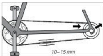
Ill.: Kædespænding (eksempel)
