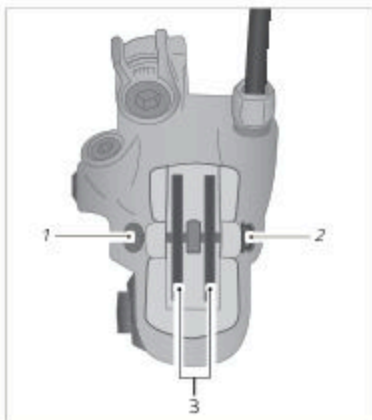
Ill.: Bremseåb med skrue (eksempel)
