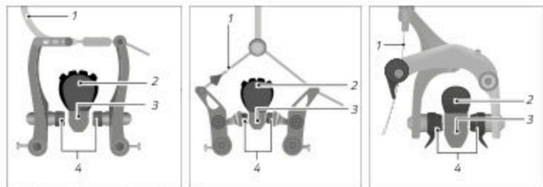
Fig: Freno de llanta mecánico (ejemplo)
