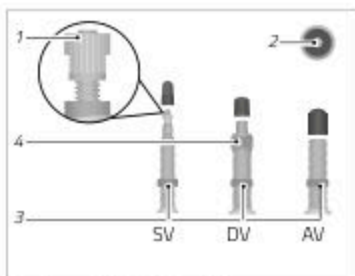
Fig.: Tipos de válvulas (ejemplo)
