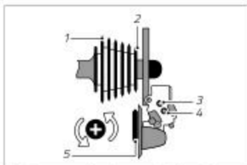
Fig.: Representación de un cambio (ejemplo)
