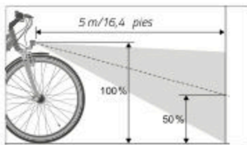
Fig.: Ajuste de la luz delantera (ejemplo)
