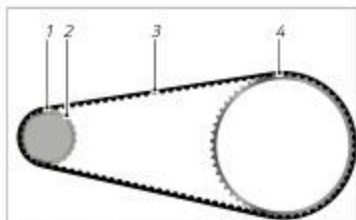
Fig.: Transmisión por correa (ejemplo)
