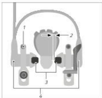
Fig: Freno de llanta hidráulico (ejemplo)
