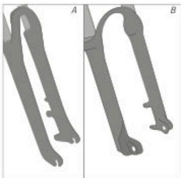
Fig: Punteras abiertas (A) y cerradas (B) (ejemplo)
