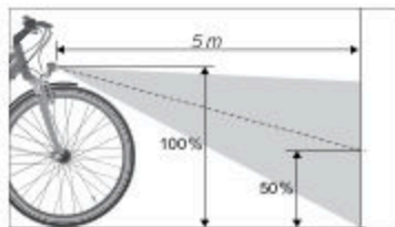
Kuva: Etuvalon säätö (esimerkki)
