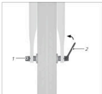
Kuva: Kiekko ja pikalukitusakseli (esimerkki)
