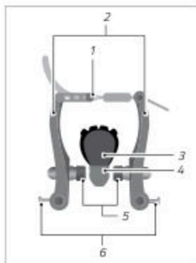
Kuva: Vannejarru ja vajerin ohjain (esimerkki)
