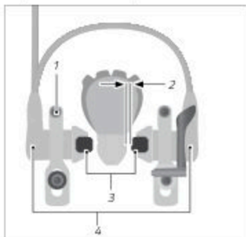
Kuva: Hydraulinen vannejarru (esimerkki)
