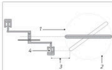
Kuva: Polkimen ja etupyörän välinen etäisyys (esimerkki)
