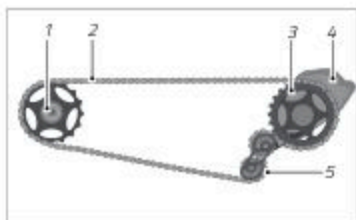
Kuva: Ketjukäytöllä varustettu Pinion-vaihteisto (esimerkki)
