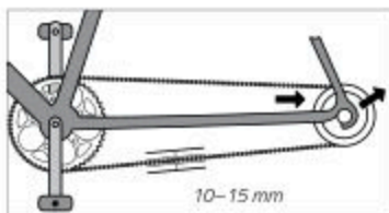
Kuva: Ketjun kireys (esimerkki)
