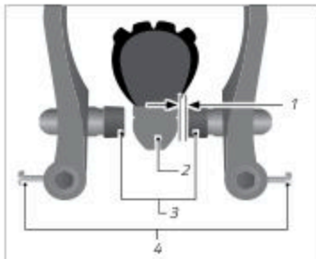
Kuva: Jarrukengän etäisyys (esimerkki)
