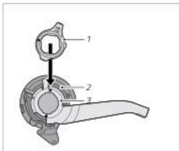
Kuva: Napavaihteiston komponentit (esimerkki)
