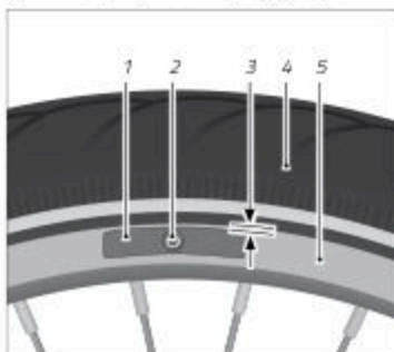
Kuva: Jarrukengän kohdistus (esimerkki)
