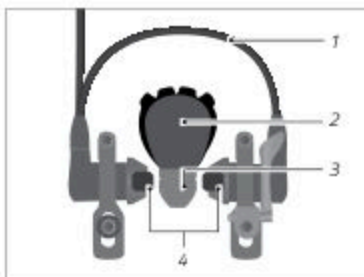
Kuva: Hydraulinen vannejarru (esimerkki)
