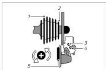
Kuva: Takavaihtajan kuvaus (esimerkki)
