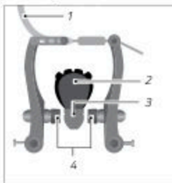
Kuva: Mekaaniset vannejarrut (esimerkki)
