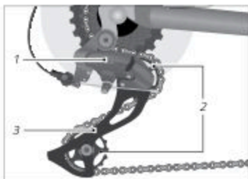
Kuva: Ketjuvaihteiston liikkuvat komponentit (esimerkki)
