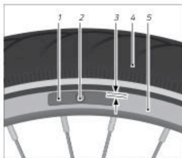
Fig. : Alignement du support de patin (exemple)
