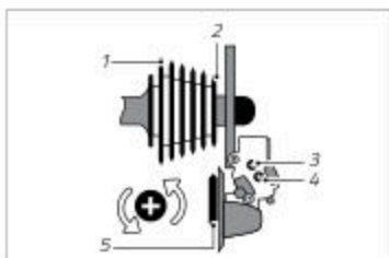
Fig. : Illustration d'un dérailleur arrière (exemple)
