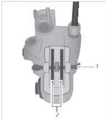
Fig. : Étrier de frein avec goupille (exemple)
