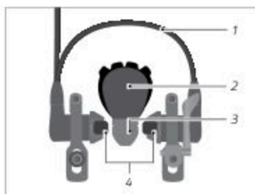
Fig. : Frein sur jante hydraulique (exemple)
