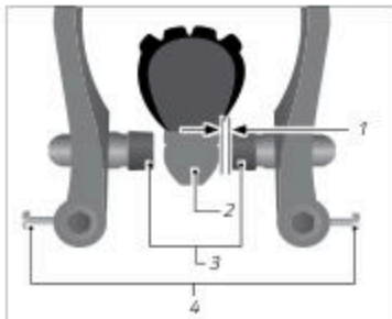
Fig. : Distance du support de patin (exemple)
