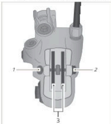
Fig. : Étrier de frein avec vis (exemple)
