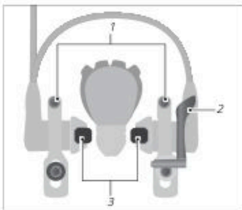
Fig. : Frein sur jante hydraulique (exemple)
