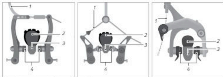
Fig. : Freins sur jante mécaniques (exemple)
