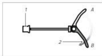
Fig : Réglage des attache rapides
