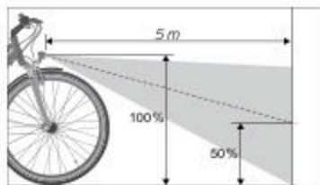
Fig. : Réglage du phare (exemple)
