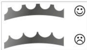
Abb.: Kettenblattverschleiß (exemplarisch)
