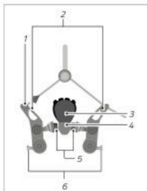
Abb.: Felgenbremse mit Seilnippel (exemplarisch)
