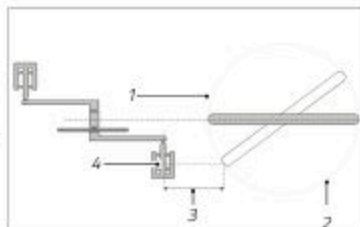
Abb.: Abstand zwischen Pedal und Vorderrad (exemplarisch)
