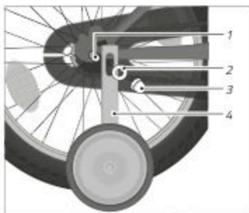
Abb.: Stützrad montieren (exemplarisch)
