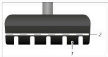
Abb.: Brems Schuh mit Verschleißindikator (exemplarisch)
