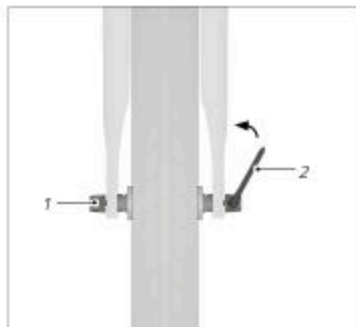
Abb.: Laufrad mit Schnellspannachse (exemplarisch)
