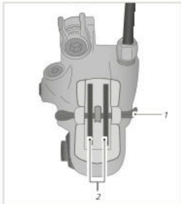
Abb.: Bremssattel mit Splint (exemplarisch)
