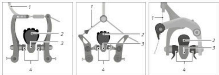
Abb.: Mechanische Felgenbremsen (exemplarisch)
