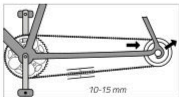
Abb.: Kettenspannung (exemplarisch)
