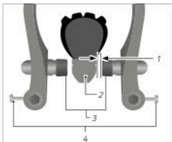
Abb.: Abstand Brems Schuh (exemplarisch)
