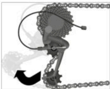
Abb.: Schaltwerk nach hinten ziehen (exemplarisch)
