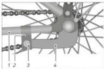
Abb.: Rücktrittbremse (exemplarisch)
