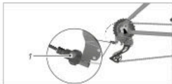
Abb.: Einstellen des Schaltwerks (exemplarisch)
