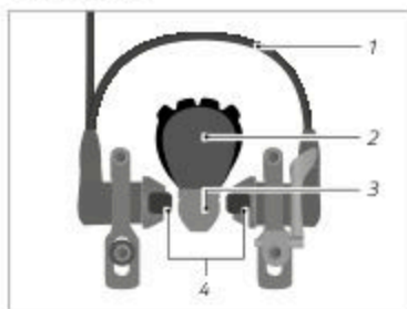
Abb.: Hydraulische Felgenbremse (exemplarisch)
