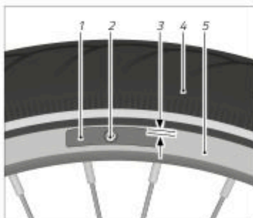
Abb.: Ausrichtung Bremsschuh (exemplarisch)
