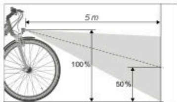
Abb.: Scheinwerfer einstellen (exemplarisch)
