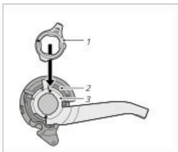
Abb.: Komponenten einer Nabenschaltung (exemplarisch)
