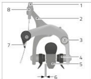
Abb.: Felgenbremse Rennrad (exemplarisch)
