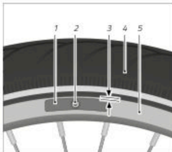
Abb.: Ausrichtung Bremsschuh (exemplarisch)
