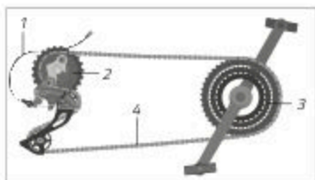
Abb.: Komponenten einer Kettenschaltung (exemplarisch)
