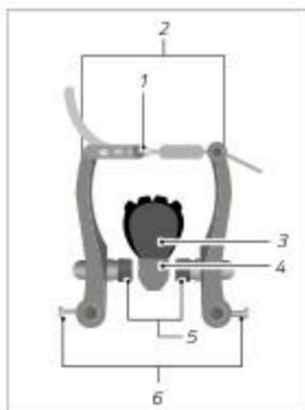
Abb.: Felgenbremse mit Zugführung (exemplarisch)
