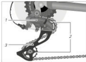
Abb.: Bewegliche Komponenten einer Kettenschaltung (exemplarisch)
