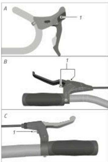
Abb.: Position Einstellschraube (exemplarisch)
