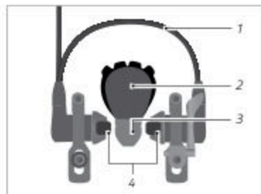
Fig: Freno a pinza idraulico (esempio)
