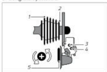
Fig.: Schema di deragliatore (esempio)
