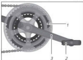
Fig: Esempio di deragliatore con cambio a 3 corone
