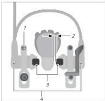
Fig.: Freno a pinza idraulico (esempio)
