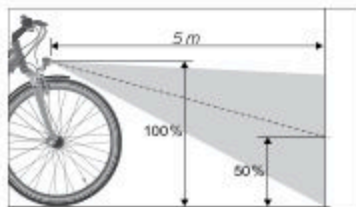
Fig.: Regolazione del fanale anteriore (esempio)
