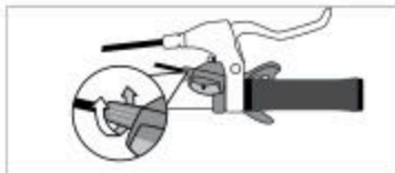
Fig.: Vite tendicavo nella leva del cambio (esempio)
