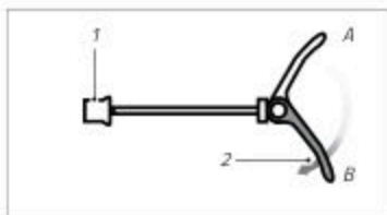
Fig. Schema dispositivo di bloccaggio a sgancio rapido (esempio)
