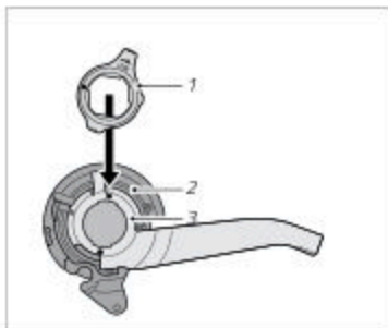
Fig.- Componenti di un cambio nel mozzo (esempio)
