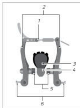
Fig: Freno a pinza con passacavo (esempio)
