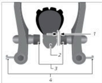
Fig.: Distanza pattino del freno (esempio)
