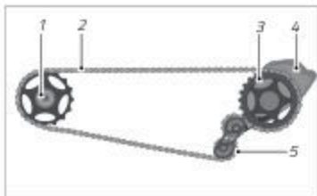
Fig: Cambio Pinion con trazione a catena (esempio)
