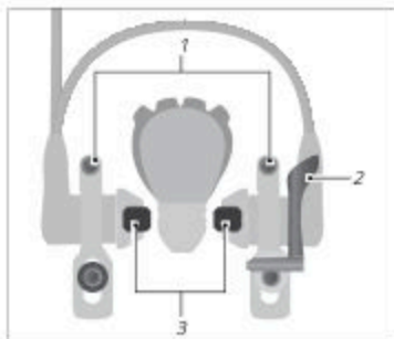
Fig.: Freno a pinza idraulico (esempio)
