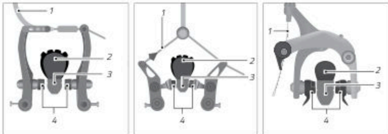
Fig.: Freni a pinza meccanici (esempio)
