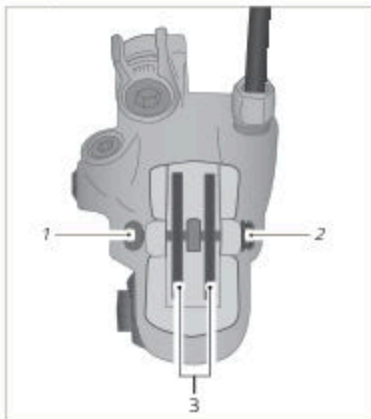
Fig: Pinza del freno con vite (esempio)
