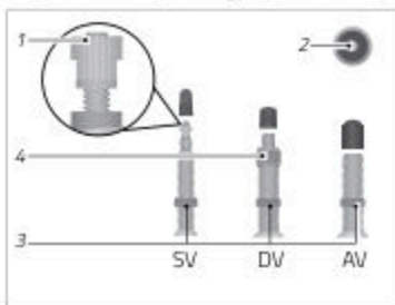
Fig.: Tipi di valvole (esempio)
