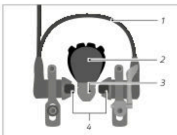
Rys: Hydrauliczny hamulec działający na obręcz koła (przykład)
