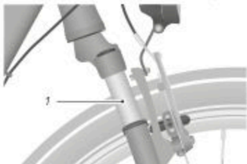
Rys.: Powierzchnia ślizgowa widełca amortyzowanego (przykład)
