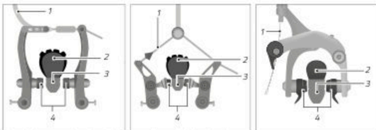
Rys: Mechaniczne hamulce działające na obręcz koła (przykład)
