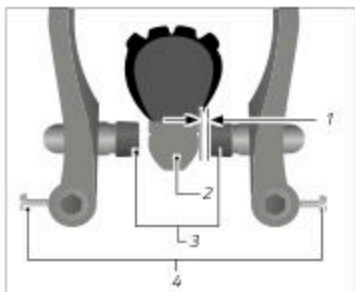
Rys.: Odstęp między klockami hamulcowymi (przykład)
