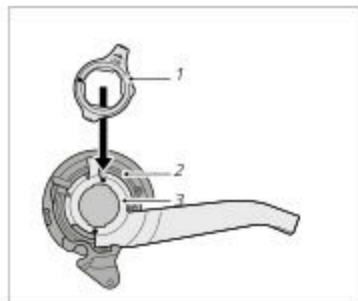
Rys.: Komponenty przerzutki wewnętrznej (przykład)
