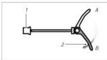
Rys.: Budowa szybkozamykacza (przykład)
