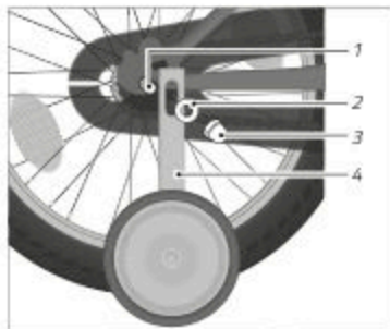
Sl.: Montaža opornega kolesa (simbolično)
