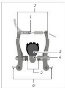
Slika: Zavora na obroču s poteznim vodilom (na podlagi primera)
