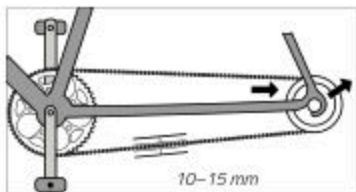
Sl.: Napetost verige (na podlagi primera)
