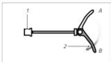
Sl: Postavitev hitrega vpenjala (na podlagi primera)
