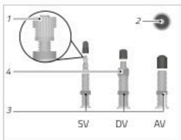
Sl: Vrste ventilov (na podlagi primera)
