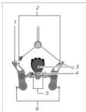
Slika: Zavora na obroču z mazalko (na podlagi primera)
