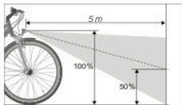
Sl.: Nastavitev žaromet (na podlagi primera)
