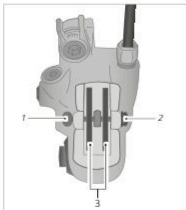
Slika: Zavorno sedlo z vijakom (na podlagi primera)
