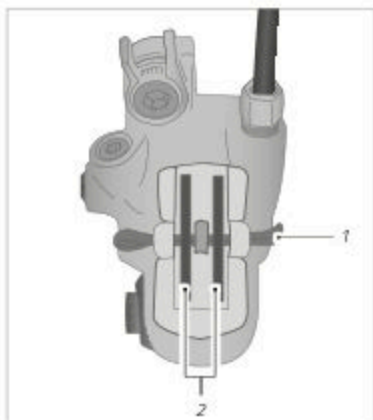
Slika: Zavorno sedlo z razcepko (na podlagi primera)
