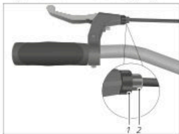
S1: Položaj protimatice in narebrčanega vijaka (na podlagi primera)
