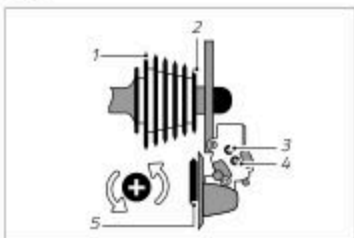
Sl.: Prikaz prestavnega mehanizma (na podlagi primera)
