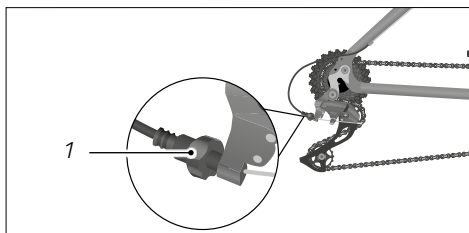
Rys.: Ustawianie tylnej przerzutki (przykład)
