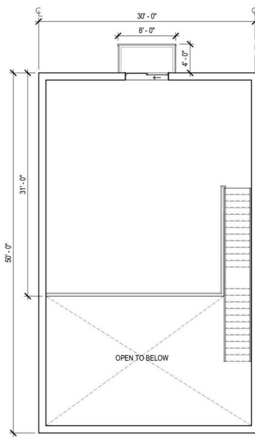
UNIT MEZZANINE 930 SF SCALE: 1/8" = 1' - 0"
