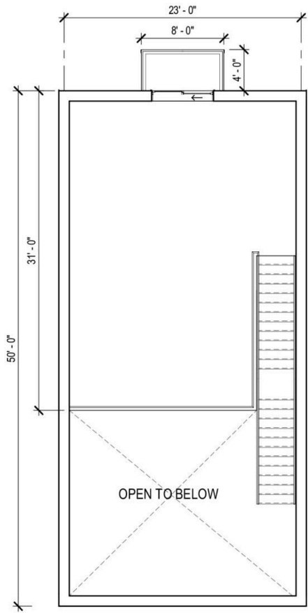
UNIT MEZZANINE 713 SF SCALE: 1/8" = 1' - 0"
