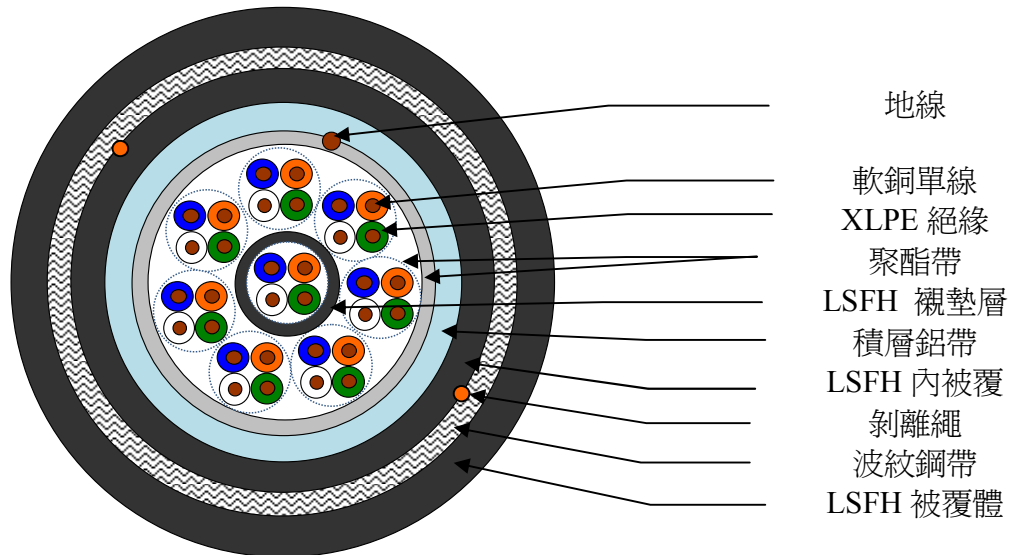
電纜構造圖
