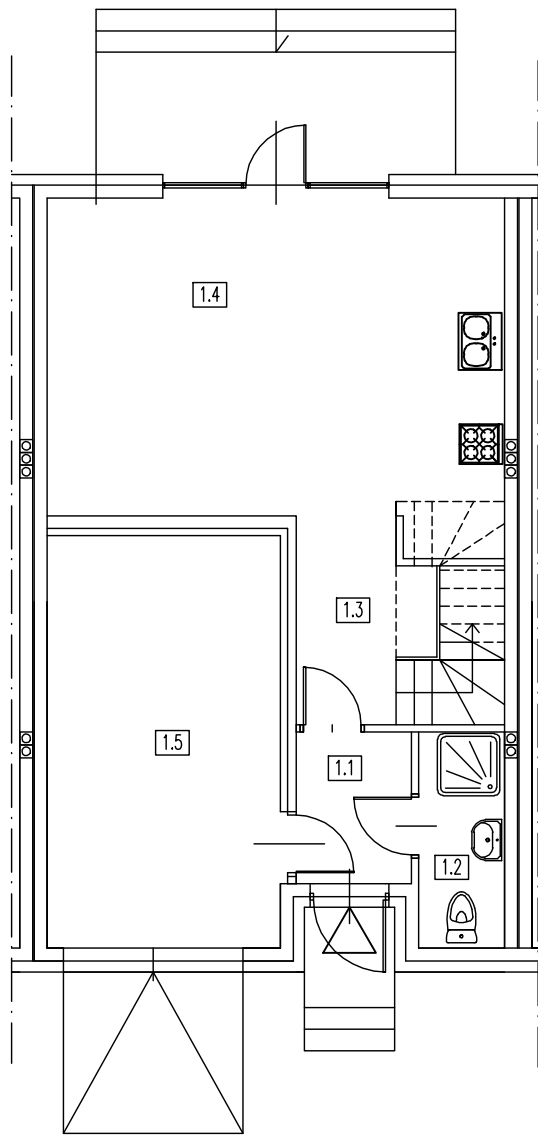
RZUT PARTERU
