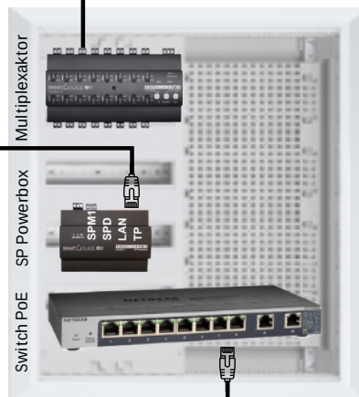
Elektroverteilung
