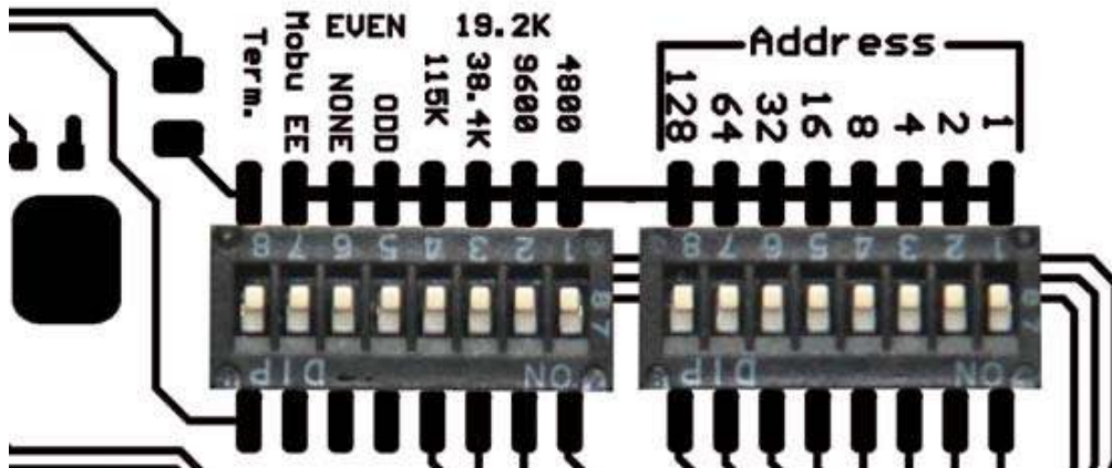
Abb. 12: Detailansicht Dipschalter
