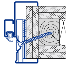
Diagonalbefestigung Montagewand F90B
