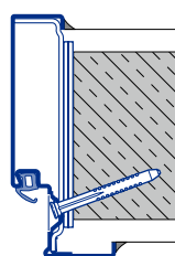
Diagonalbefestigung Sichtbeton / Sichtmauerwerk bis MW 175
