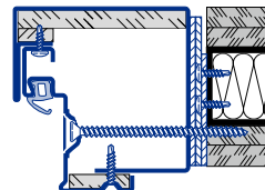
Schraubmontage Montagewand F90A
