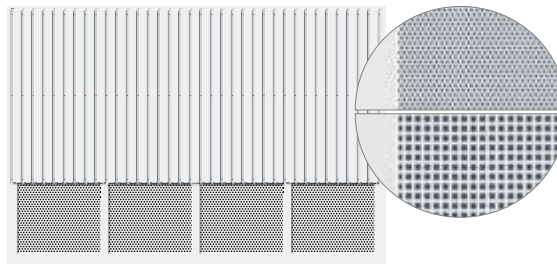
Motiv 414 Auflegendes, gesicktes Stahlblech mit Lochblechfüllung, rund oder quadratisch, Lüftungsquerschnitt 46,1% (rund) bzw. 44,4% (quadratisch)
