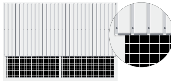
NEU. Motiv 416 (ET 450) Auflegendes, gesicktes Stahlblech mit Gitterfüllung 50 × 50 mm im unteren oder oberen Bereich (Abb. zeigt unteren Bereich), Lüftungsquerschnitt 23,2%
