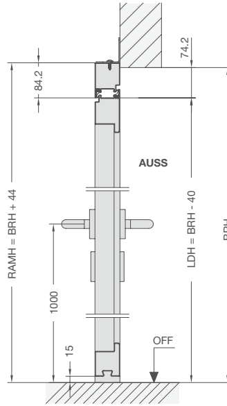
Vertikalschnitt
