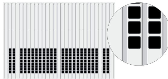
NEU. Motiv 414 (ET 450) Auflegendes, gesicktes Stahlblech mit Quadratlochung 50 × 50 mm im unteren oder oberen Bereich (Abb. zeigt unteren Bereich), Lüftungsquerschnitt 11,5%.
