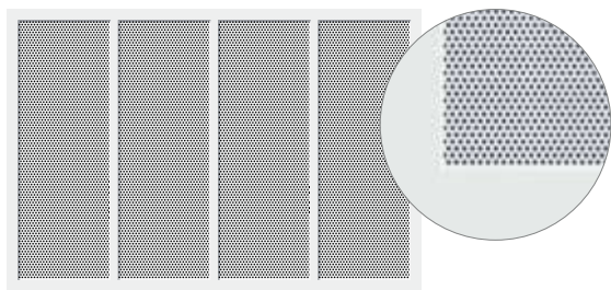
Motiv 412 und 432 Innenliegende Lochblechfüllung (Motiv 412 Stahl-Lochblech, Motiv 432 Aluminium-Lochblech) mit runden Aussparungen, Lüftungsquerschnitt 46,1%
