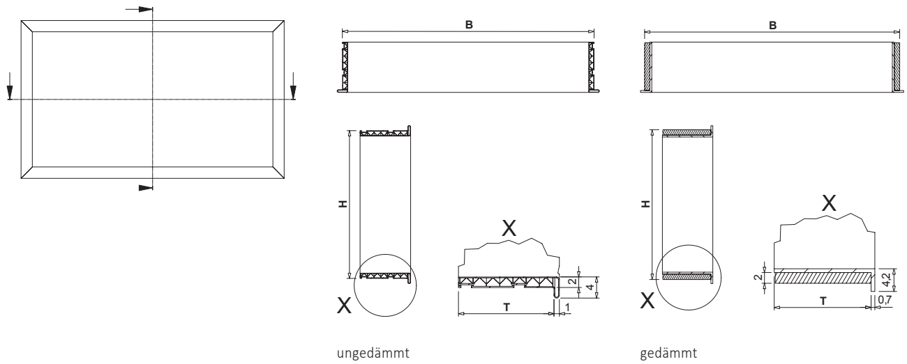
Maßtabelle MEAFRAME, 1-teilig, für MEALUXIT / MEATHERMO
