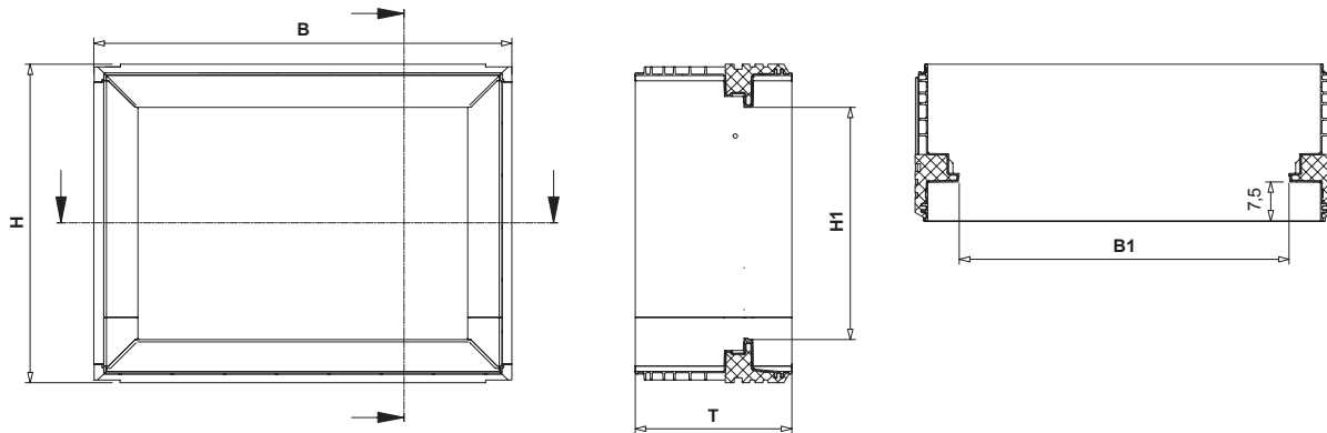
Maßtabelle Zarge MEALUXIT
