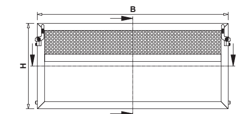
MEALUXIT Kipp E mit Lüftungseinsatz (Maße in cm)
