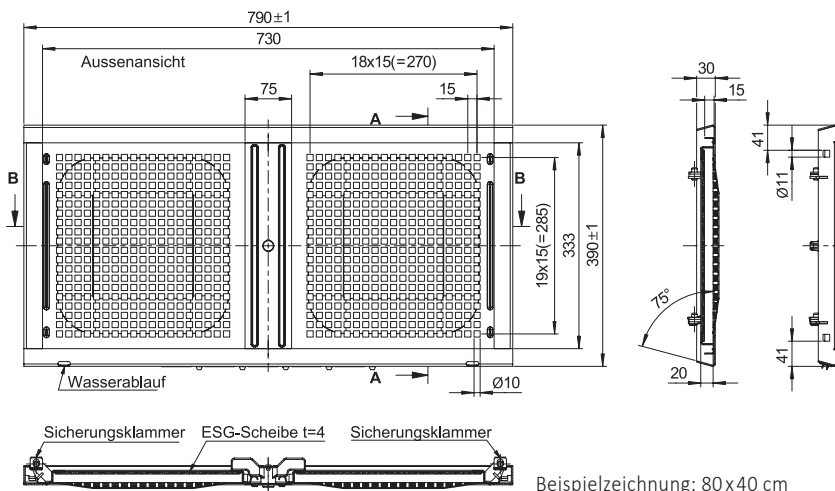
Maßtabelle MEALIT 2-flüglig mit festem Mittelstück
