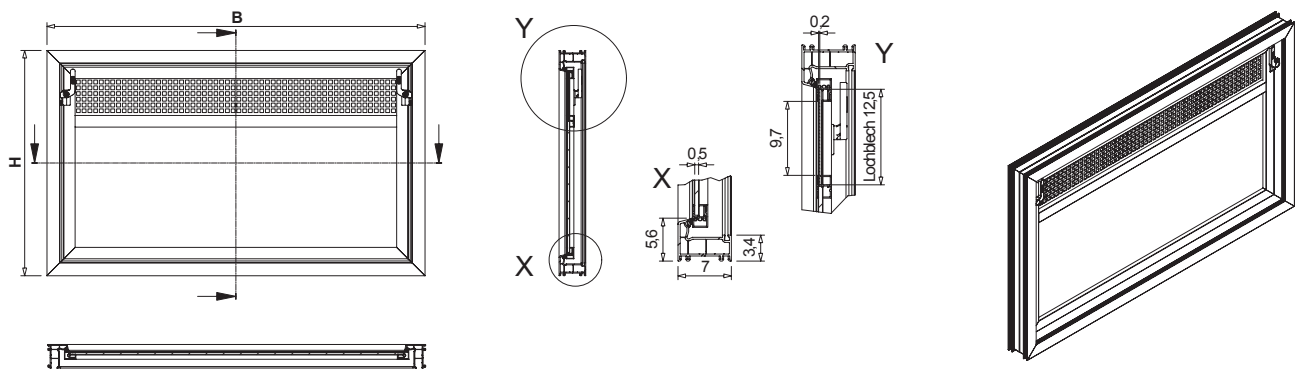
MEALON Kipp E mit Lüftungseinsatz
