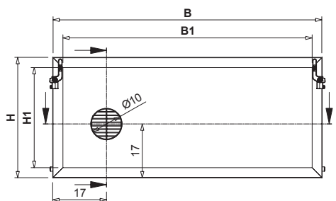
MEALUXIT Kipp E mit Abluftanschluss (Maße in cm)
