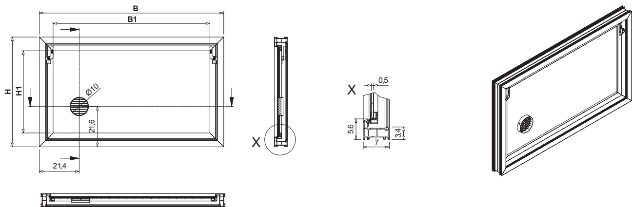
MEALON Kipp E mit Lüftungseinsatz
