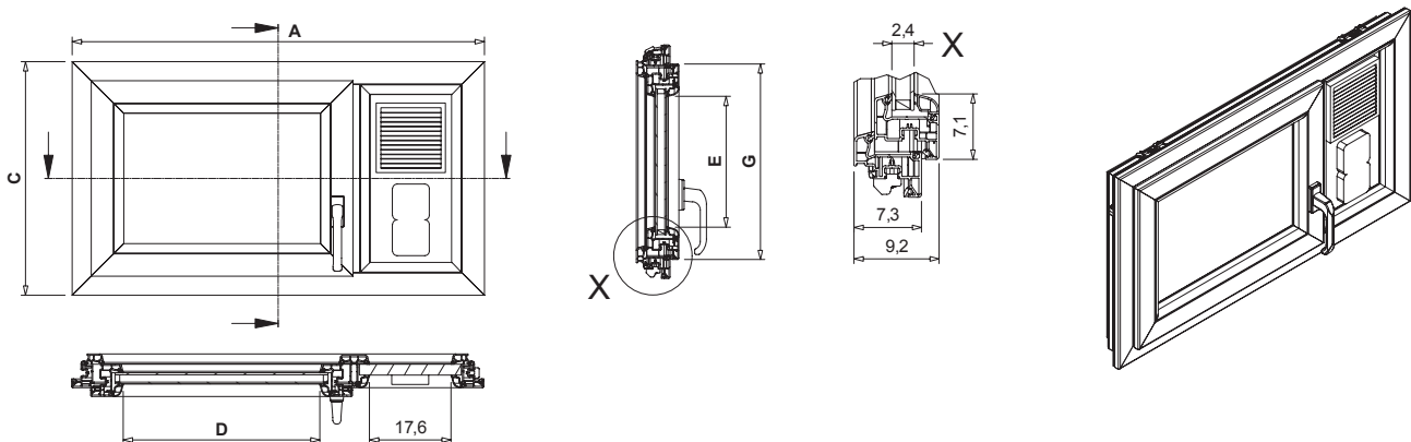
Maßtabelle Fenstereinsatz MEALUXIT mit MEALÜFT AIR
