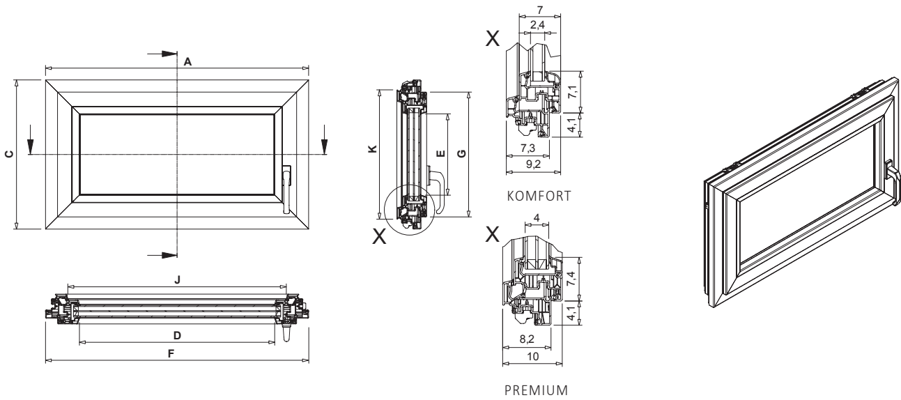
Maßtabelle Fenstereinsatz MEALUXIT Dreh-Kipp KOMFORT/PREMIUM
