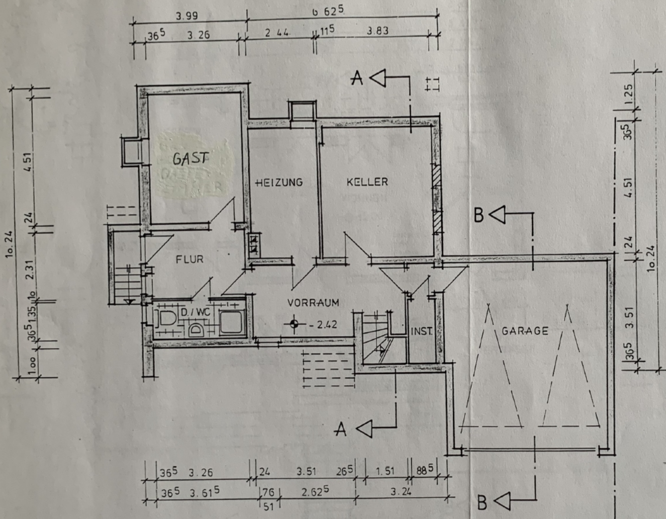
KELLERGESCHOSS M 1:100
