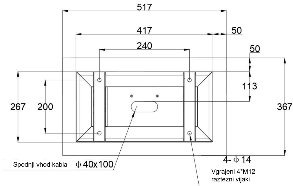
Slika 6-2-2 Način namestitve tipa za namestitev na tla
