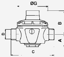
Type 9 male/male
