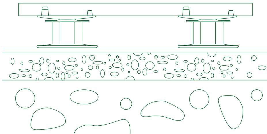
Verdichtetes Schotterbett
